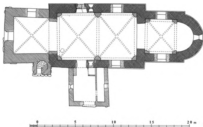
Fig. 2. Plan. 1:300. Målt af MB 1966, tegnet af Marianne Nielsen 1984. Signaturforklaring s. 9. - Ground-plan. Key on p. 9.
