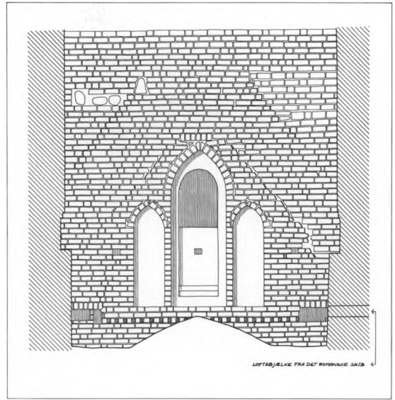
Fig. 5. Vestforlængelsens gavl med skrå taglinjer (s. 1118) og forhøjelsens kam, afsluttet af musetrapper (s. 1121). 1:100. Målt af HeJ og tegnet af Marianne Nielsen 1984. - Gable of the west extension.
