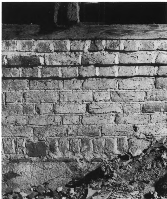
Fig. 7. Skibets oprindelige murkrone med forhøjelsen i forbindelse med hvælvslagningen, set fra nordkapellets loft (s. 1118, 1121). HJ fot. 1984. - The nave's original walls heightened for the vaults, seen from the loft of the north chapel.
