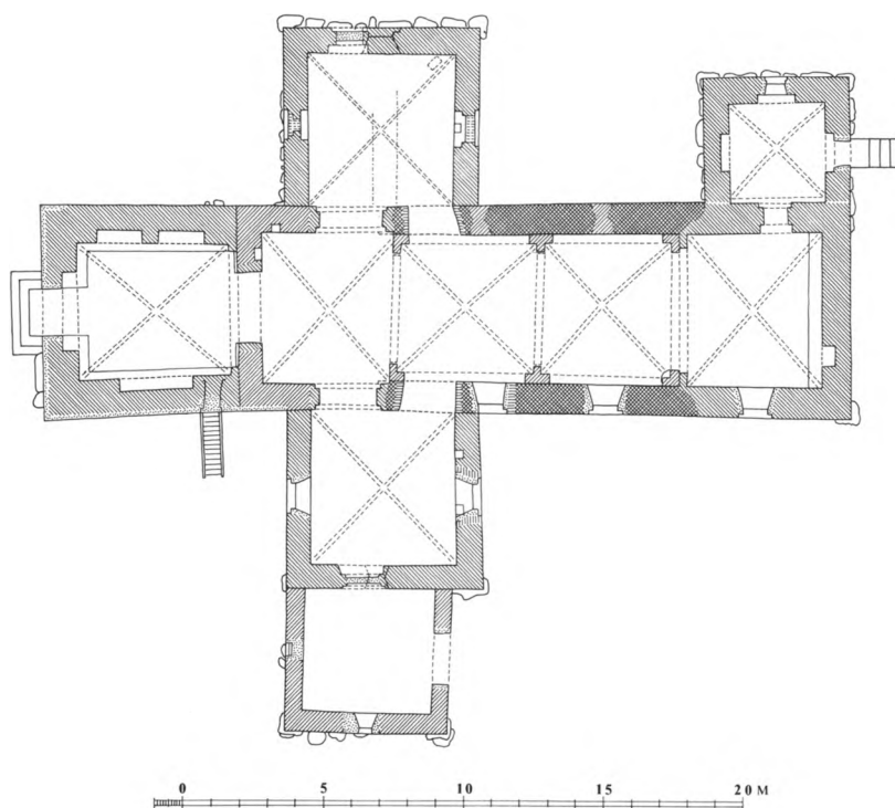
Fig. 4. Plan. 1:300. Målt af HeJ og HJ 1982, tegnet af Marianne Nielsen 1984. Signaturforklaring s. 9. - Ground-plan. Key on p.9.
