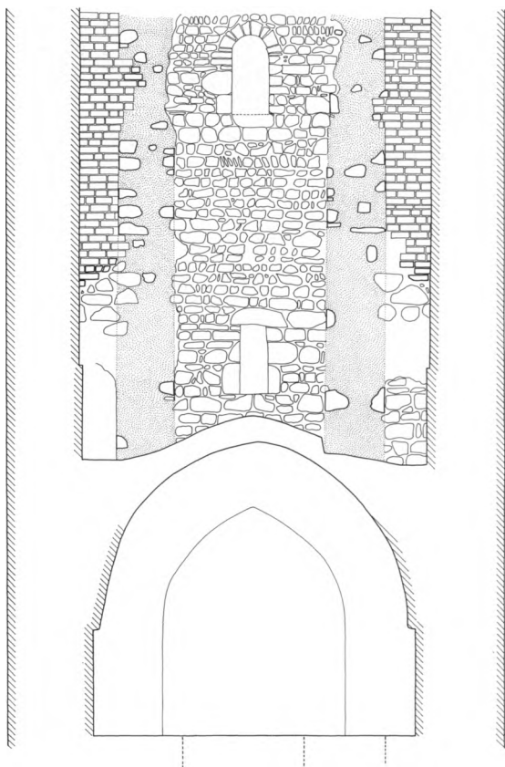
Fig. 3. Tværnsnit i tårnet, set mod skibets gavl med rester af (†)romansk tårn, jfr. fig. 4 og 5 (s. 1184). 1:100. Målt af HeJ og tegnet af Marianne Nielsen 1984. - Cross-section of the tower, looking towards the nave gable with the remains of the Romanesque (†)tower, cf. figs- 4 & 5.
