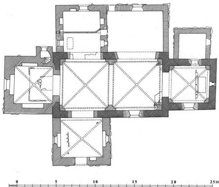
Fig. 2. Plan. 1:300. Målt af C. G. Schultz 1938, suppleret af HS 1964, KdeFL 1965 og tegnet af Marianne Nielsen med revisioner 1984. Signaturforklaring s. 9. - Ground-plan. Key on p. 9.
