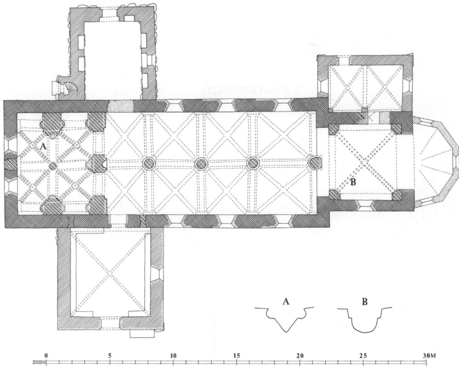
Fig. 6. Plan. 1:300. Målt af HeJ 1983, tegnet af Marianne Nielsen 1986. Signaturforklaring s. 9. - Ground-plan. Key on p. 9.
