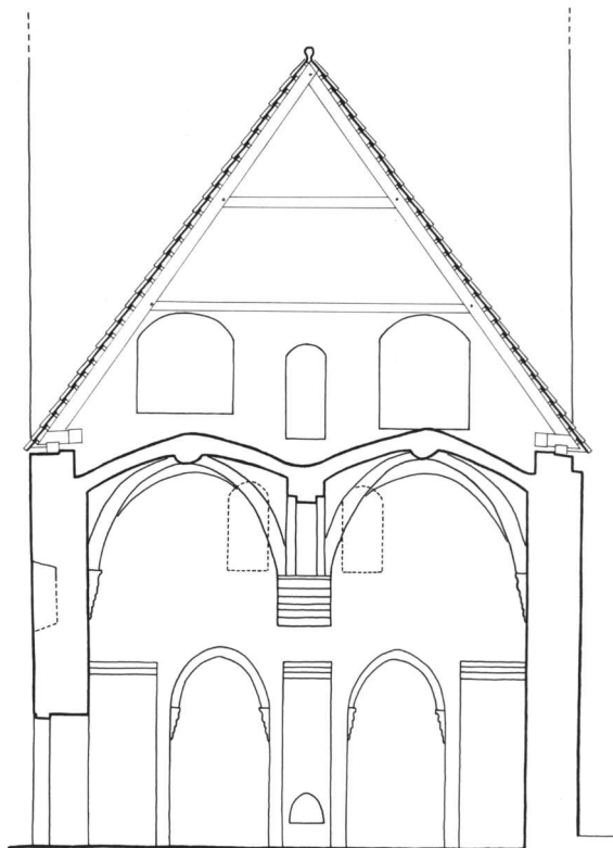
Fig. 19. Tværnsnit. 1:150. Målt af Hej 1983, tegnet af Marianne Nielsen 1986. - Cross-section.
