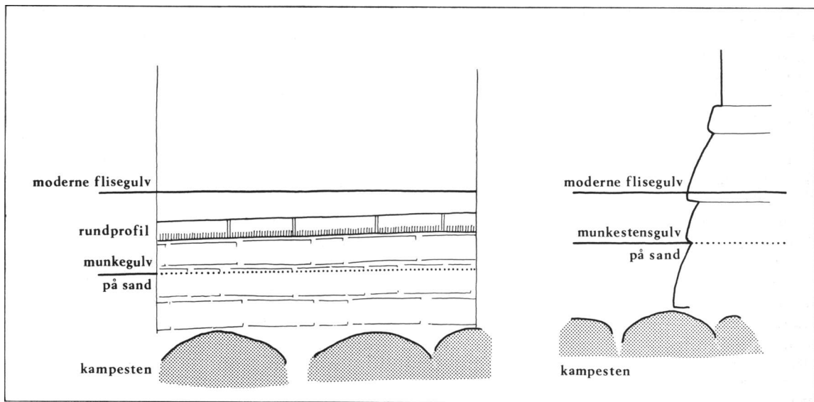
Fig. 51a-b. (†)Detaljer af kirkens senromanske ombygning: a. Facade af sokkel på tårnskillevæggens nordre lisen (s. 1551). b. Snit af base på skibets vestligste rundpille (s. 1548). 1:20. Tegnet af Marianne Nielsen 1987 efter skitse ved Chr. Axel Jensen 1918. - 51a-b. (†)Details of the late Romanesque alterations: a. Facade on base of lesene to the north on the partition wall of the tower. b. Section of base of the westernmost column in the nave.
