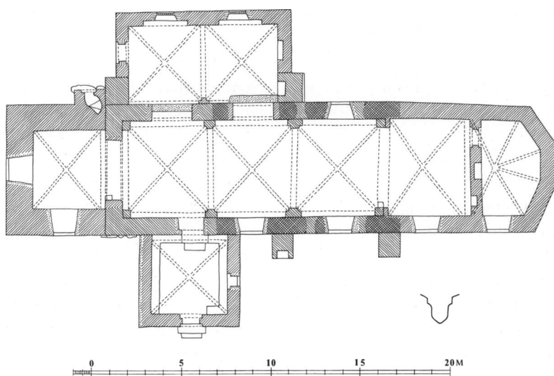
Fig. 3. Plan. 1:300. Målt af Charles Christensen 1921, tegnet af Marianne Nielsen 1987. Signaturforklaring s. 9. - Ground-plan . Key on p. 9.
