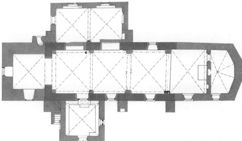
Fig. 11. Plan. 1:300. Tegnet af J. B. Løffler 1881. NM2. - Ground-plan.
