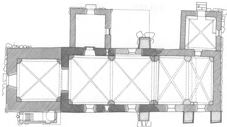
Fig. 3. Plan. 1:300. Målt af Aage Herløw 1926 og tegnet af Marianne Nielsen 1987. Signaturforklaring s. 9. - Ground-plan. Key on p. 9.
