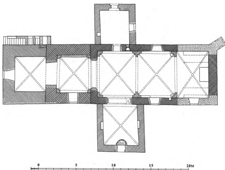
Fig. 2. Plan. 1:300. Målt af Aage Herløw, suppleret 1958 og tegnet 1988 af Marianne Nielsen. Signaturforklaring s. 9. - Ground-plan. Key on p. 9.
