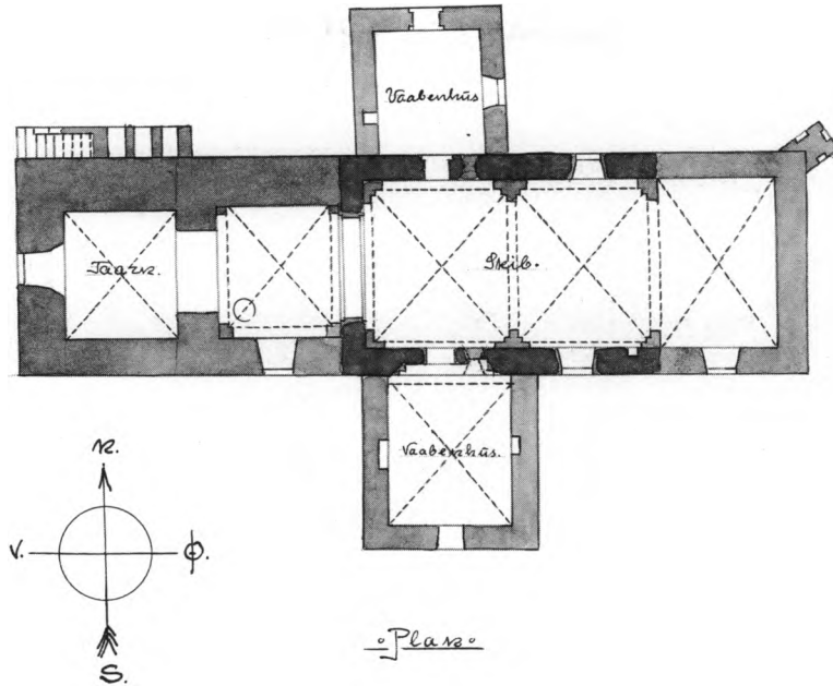
Fig. 3. Plan. 1:300. Målt af Aage H. Mathiesen 1895. - Ground-plan.
