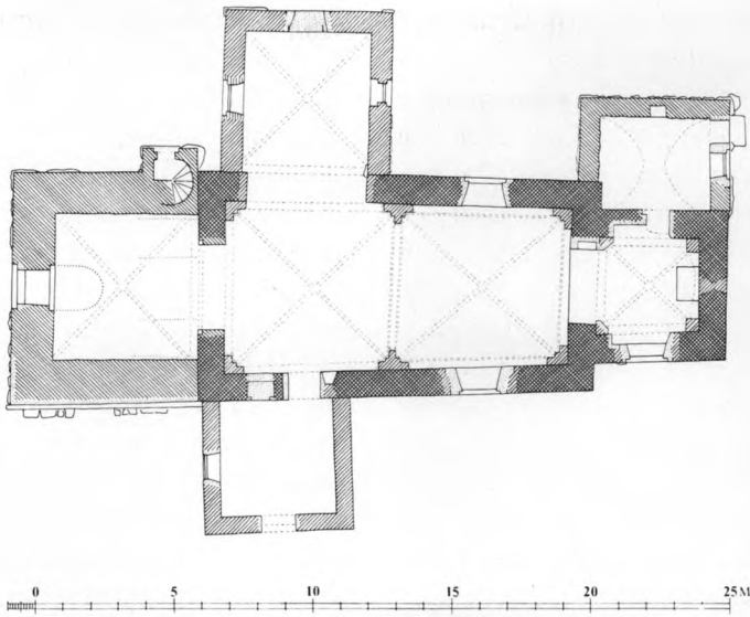
Fig. 3. Plan. 1:300. Målt af Per Godtfredsen 1966, suppleret af Birgit Als Hansen 1982 og tegnet af Marianne Nielsen 1989. Signaturforklaring s. 9. - Ground-plan. Key on p. 9.
