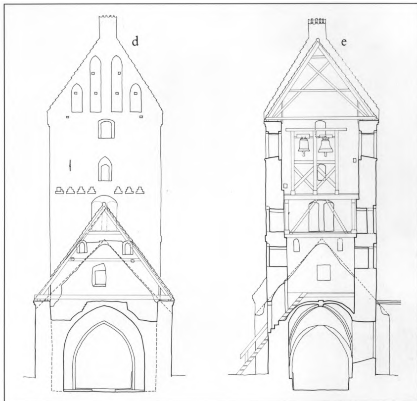
Fig. 7a-e. Opmålinger af tårn 1:200. a. Nordfacade. b. Vestfacade, c. Sydfacade, d. Østfacade over tværnsnit i skib. e. Tværnsnit, set mod øst. Målt og tegnet af Peter Kristiansen 1989, delvis på grundlag af opmålinger i Marinus Andersens arkiv. - Measured drawings of tower 1:200. a. North facade, b. West facade, c. South facade, d. East facade above cross-section of nave. e. Cross-section looking east.
