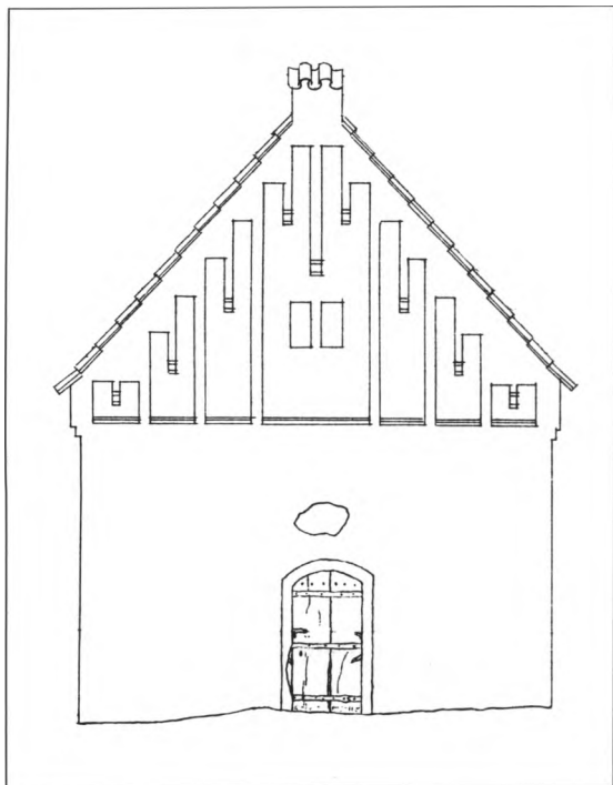
Fig. 11. Nordkapellets gavl (s. 1970). 1:100. Udsnit af kirkens nordfacade, målt af Mogens Biilmann, Chr. Olrik og H. Schønnemann. Marinus Andersens arkiv. - Gable of the north chapel. Detail of the church's north facade.
