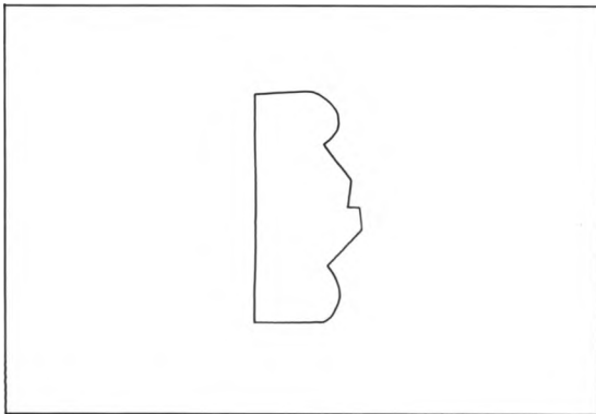
Fig. 15. Formsten til vinduesfals (s. 1973). 1:10. Målt af EIM 1966 og tegnet af Marianne Nielsen 1989. - Moulded brick for window.
