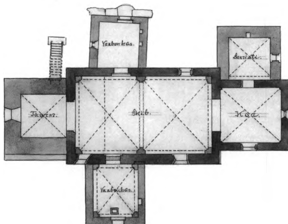
Fig. 21. Plan. 1:300. Målt og tegnet af Aage H. Mathiesen 1895. - Ground-plan.
