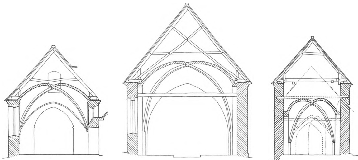
Fig. 5a-c. Tværsnit. 1:150. a. Kor, set mod vest. b. Skib, set mod vest. c. Sydkapel, set mod nord. Målt og tegnet af Jan Gehl 1963; dog er fig. 5a og c suppleret og omtegnet ved Marianne Nielsen 1989. - Cross-sections. 1:150. a. Chancel seen to the west. b. Nave seen to the west. c. South chapel seen to the north.
