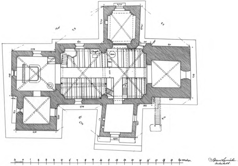
Fig. 53. Plan. 1:300. Målt og tegnet af Søren Lemche 1919. Syd opad. - Ground-plan. (South up).
