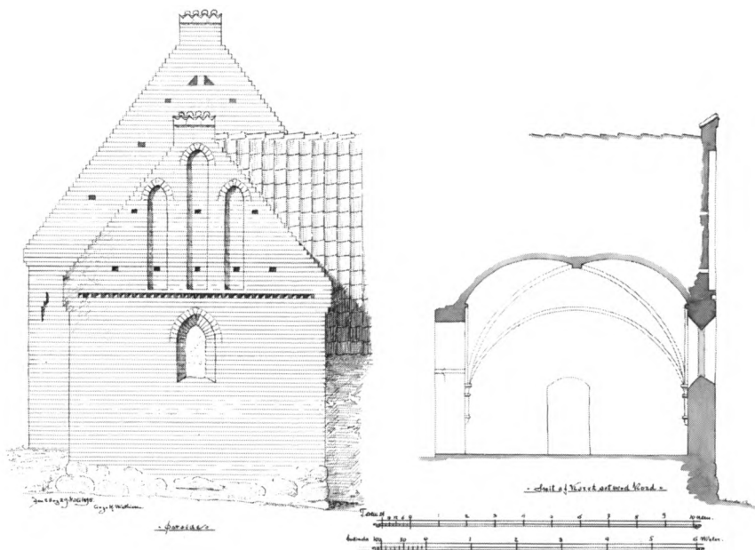
Fig. 8. Facade mod øst og længdesnit i kor, set mod nord. 1:150. Målt og tegnet af Aage H. Mathiesen 1895. - Facade to the east and longitudinal section of the chancel seen to the north.
