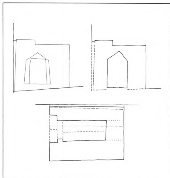
Fig. 32. Middelalderligt alterbord. 1:50. Opstalt af nordsiden, snit set mod syd og plan. Målt og tegnet af Peter Kristiansen 1989 (s. 2020). - Medieval altar. Elevation, section and plan.
