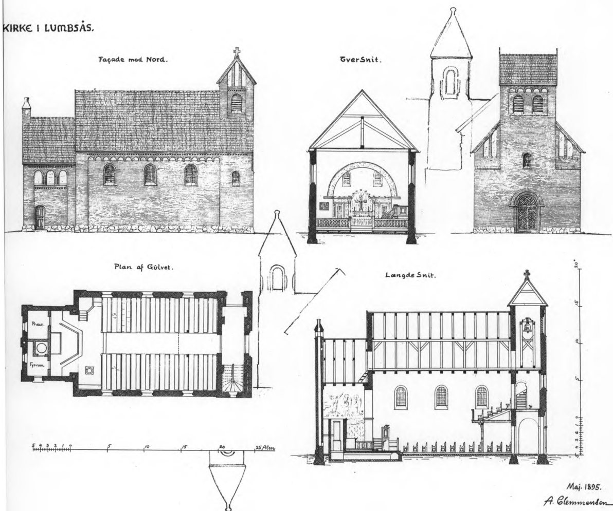
Fig. 1. Plan, snit og facader ved Andreas Clemmensen, maj 1895. 1:300. På bladet er med blyant skitseret tårnet til kirken i Lynæs, tegnet af samme arkitekt få år senere, jfr. DK. Frborg, s. 1670. Kunstakademiets Bibliotek. - Ground-plan, sections and facades by Andreas Clemmensen, may 1895. On the sheet is sketched the outline of the tower for the church in Lynæs, drawn by the same architect a few years later.
