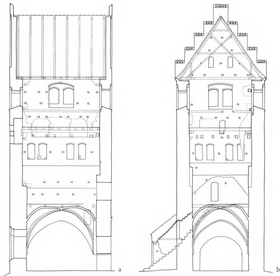
Fig. 13a-b. Snit i tårn. 1:200. a. Øst-vest. b. Nord-syd. Målt og tegnet af Peter Kristiansen 1990, til dels på grundlag af opmåling ved K. Sørensen og L. Bahn 1986. - a-b. Sections of the tower, a. East-west. b. North-south.
