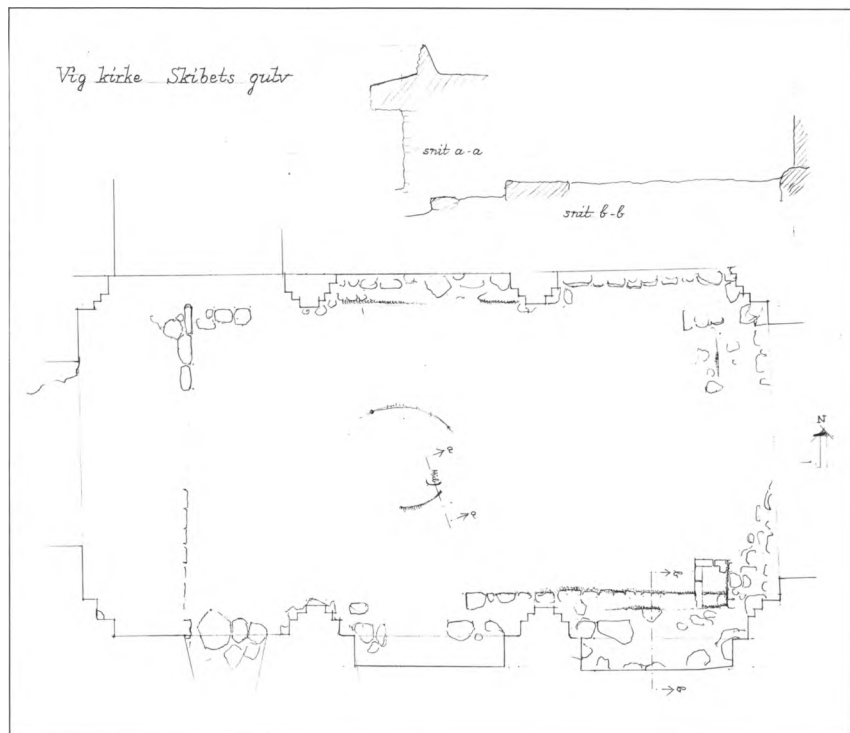
Fig. 9. Udgravning i skibets gulv med levn af sidealterborde (s. 2219), fontepodium (s. 2225), vægbænke og kirkeejersplads i vestenden (s. 2217). Plan 1:150, snit 1:30. Tegnet af Aage Roussell 1960. - Excavation of the nave floor with remains of side altars, font podium, walled benches and church patron's podium in the west end.
