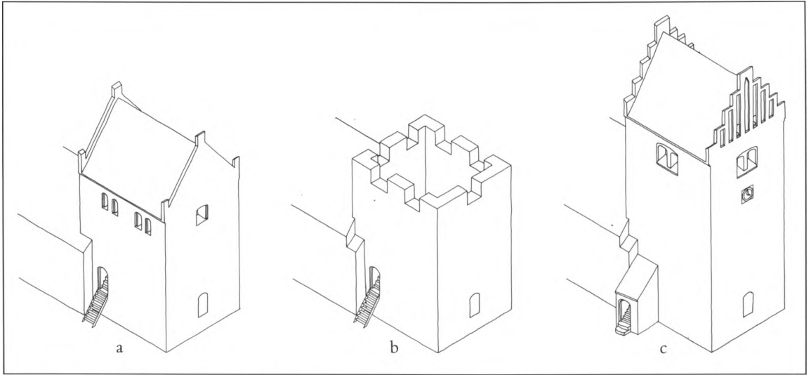
Fig. 12a-c. Isometriske rekonstruktioner af tårnets bygningshistorie (s.2209f.). 1:300. Peter Kristiansen 1990. a. Det ældste tårn o. 1400. b. Første projekt til en forhøjelse, c. Det forhøjede tårn fra 1490'erne. - a-c. Isometric reconstruction of the tower's building history, a. The earliest tower c. 1400. b. The first project for a heightened tower. c. The heightened tower from the 1490s.
