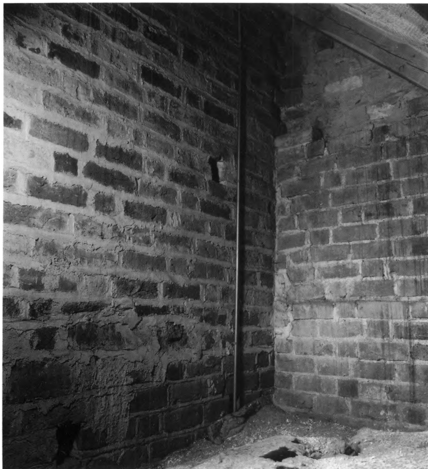
Fig. 18. Detalje af korets nordmur, set fra sakristiets loft. Foruden ses rest af det omhyggeligt fugede senromanske murværk (s. 2207), hvorover det skødesløse murværk fra korets senmiddelalderlige ombygning med fortanding til sakristiets gavl (s. 2213f.). HJ fot. 1990. - Detail of the chancel's north wall seen from the sacristy loft. Below is a relic of the meticulously laid late Romanesque brickwork, above which is the careless walling from the late medieval rebuilding of the chancel with toothing for the sacristy gable.
