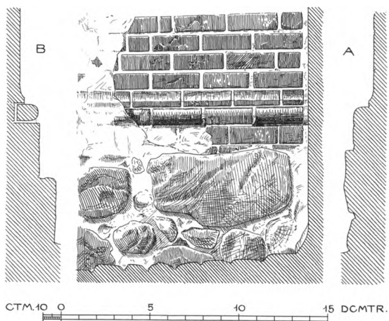
Fig. 10. Levn af sokkel på nordsiden af senromansk kor. Facade samt oprindelig (A) og sekundær (B) profil. 1:30. Målt og tegnet af C. G. Schultz 1929. - Relics of the plinth on the north side of the late Romanesque chancel. Facade, as well as the original (A) and secondary (B) mouldings.
