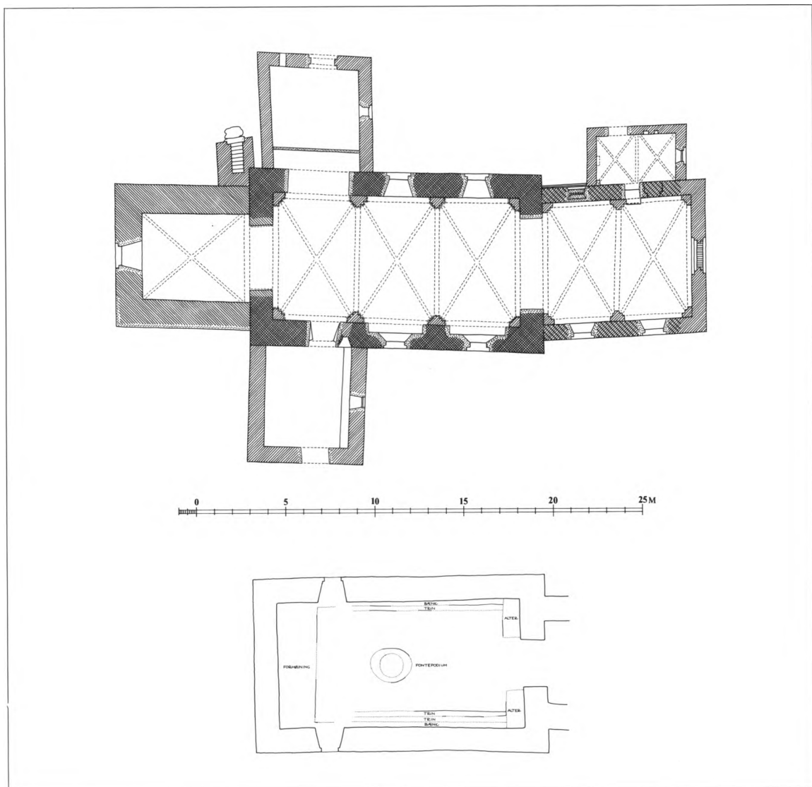
Fig. 7-8. Planer. 1:300. 7. Kirken, målt af C. G. Schultz 1929, suppleret af HJ 1982 og tegnet af Marianne Nielsen 1991. Signaturforklaring s. 9. 8. Skibets oprindelige indretning. Rekonstruktion ved Olaf Olsen på grundlag af fig. 9. Tegnet af Morten Aaman Sørensen 1966. - Ground-plans. 7. The church. Key on p. 9. 8. The original arrangement in the nave. Reconstruction by Olaf Olsen on the basis of fig. 9.
