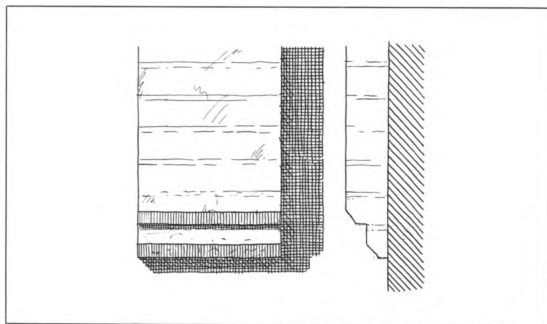
Fig. 50. †Murfremspring på indersiden af sakristiets vestgavl (s. 2215). 1:25. Målt og tegnet af C. G. Schultz 1929. — †Wall projection on the inner face of the west gable of the sacristy.
