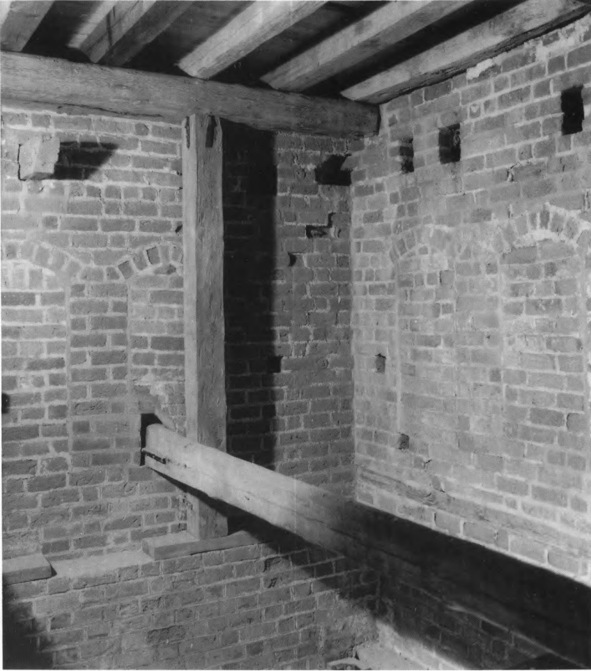
Fig. 14. Nord- og østsiden af tårnets mellemstokværk med blændede glamhuller fra det ældste, lave tårn (s. 2210). HJ fot. 1990. - North and east face of the tower's middle storey with walled up belfry lights of the low earliest tower.
