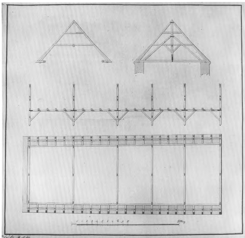
Fig. 14. Plan og snit af nyt tagværk til langhuset, udfærdiget 1824 af kgl. bygningsinspektør Peter Krogh Bonsach Jessen (s. 2290). Rigsarkivet. - Plan and sections of new roof construction over the nave prepared in 1824 by Peter Krogh Bonsach Jessen, H.M. Inspector of Buildings.
