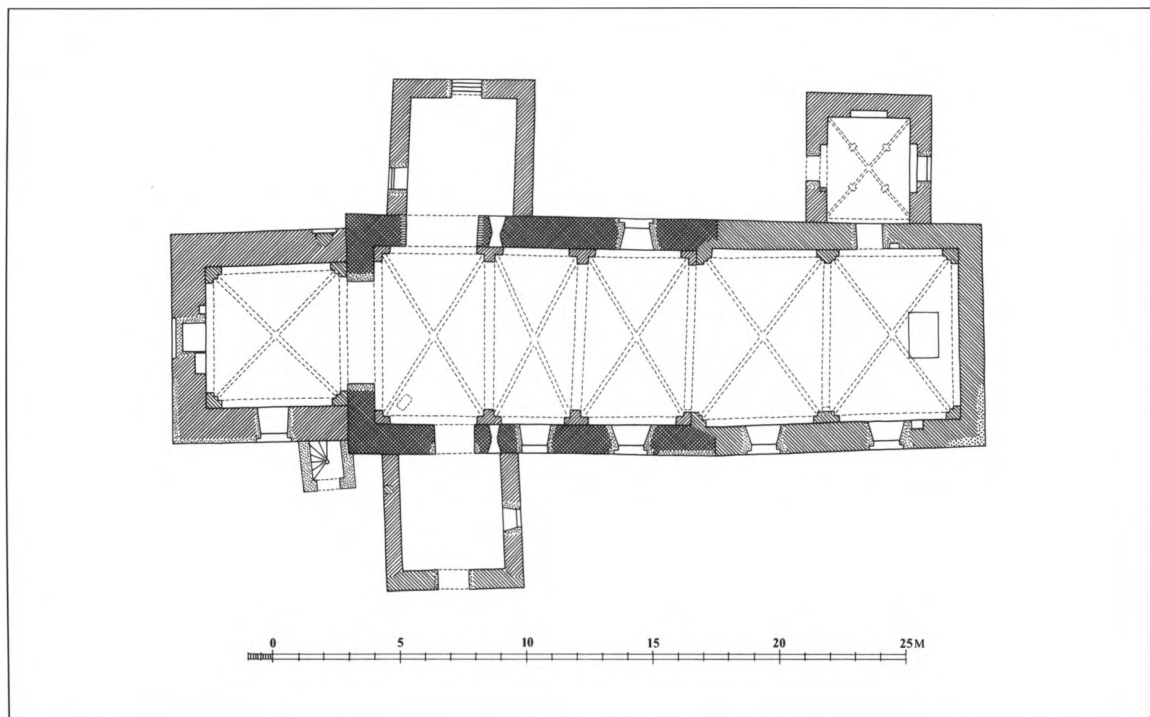
Fig. 5. Plan. 1:300. Målt af C. G. Schultz 1929, revideret af HJ 1981 og tegnet af Marianne Nielsen 1991. Signaturforklaring s. 9. - Ground-plan. Key on p. 9.
