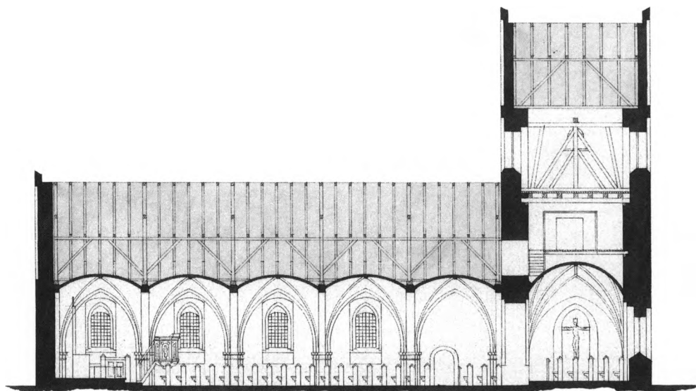
Fig. 5b. Længdesnit, set mod syd. Jfr. fig. 5a. - Longitudinal section looking south.
