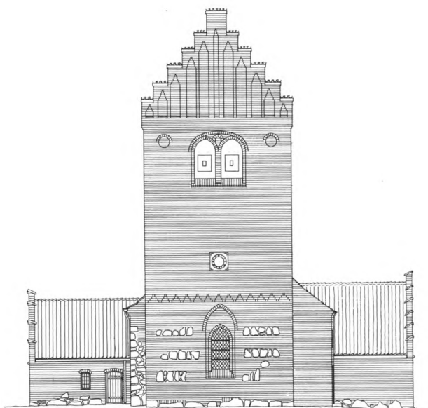
Fig. 7a-c. Opmålinger. 1:300. a. Sydfacade. b. Vestfacade. c. Længdesnit, set mod nord. Målt af C. G. Schultz 1926. - a-c. Elevations a. South facade. b. West facade. c. Longitudinal section looking north.
