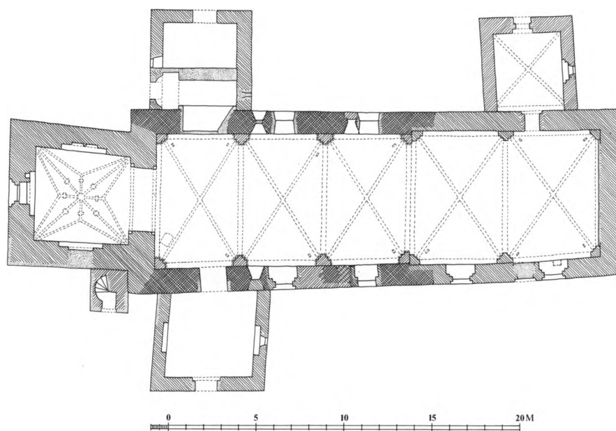
Fig. 4. Plan. 1:300. Målt af C. G. Schultz 1929, tegnet og suppleret af Mogens Vedsø 1991. Signaturforklaring s. 9. - Ground-plan. Key onp. 9.
