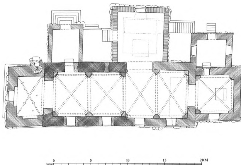
Fig. 4. Plan. 1:300. Målt af C. G. Schultz 1929, tegnet og suppleret af Mogens Vedsø 1992. Signaturforklaring s. 9. - Ground-plan. Key on p. 9.
