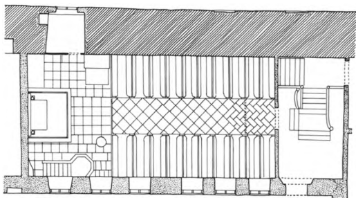
Fig. 3. Plan. 1:300. Målt af Emil Jørgensen 1908, Tegnet af Mogens Vedsø 1992. Signaturforklaring s. 9. - Ground-plan. Key on p.9.
