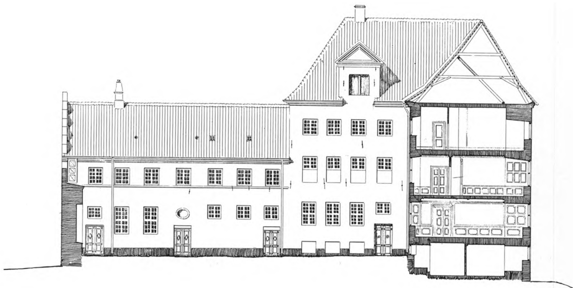
Fig. 2a-b. Opmålinger. 1:300. a. Nordfløjens gårdfacade, b. Østfløjens gårdfacade med tværsnit gennem kapellet. Målt af Emil Jørgensen 1908. - Elevations, a. North wing cross-section through the chapel. b. East wing, courtyard facade with cross-section through the chapel.
