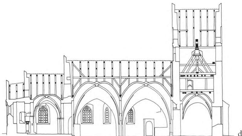
Fig. 6a-d. Opmålinger. 1:300. a. Tværnsnit i kor set mod øst. b. Tværnsnit i skib set mod øst. c. Tværnsnit i skib set mod vest. d. Længdesnit set mod syd. Sammentegnet af Mogens Vedso 1992 på grundlag af opmålinger ved Aage Mathiesen 1895, Anders P. Pedersen og Th. Mortensen 1911, Marinus Andersen o. 1948 og Hej 1976. - Elevations. 1:300. a. Cross-section of chancel to the east. b. Cross-section of nave to the east. c. Cross-section of nave to the west. d. Longitudinal section to the south.
