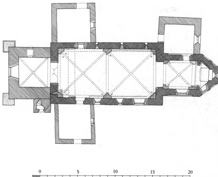
Fig. 4. Plan. 1:300. Målt af C. G. Schultz 1992, tegnet og suppleret af Mogens Vedsø 1992. Signaturforklaring s. 9. - Ground-plan. Key on p.9.
