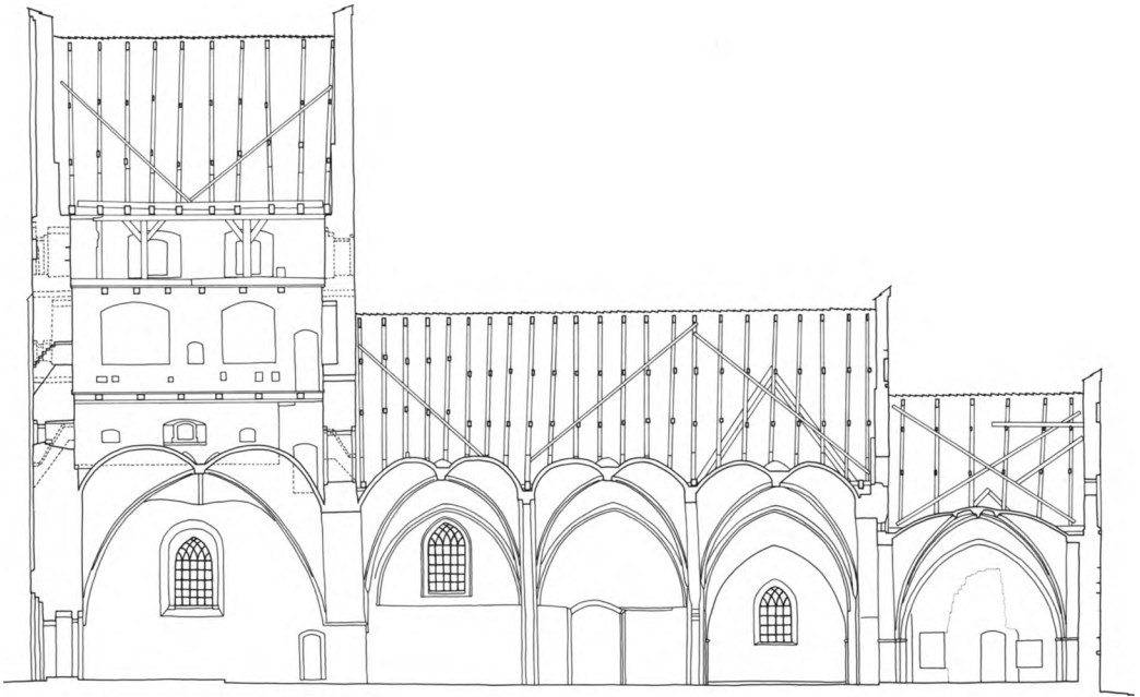
Fig. 7. Længdesnit. 1:300. Målt og tegnet af Mogens Vedsø 1989 og 1991. Tagværkerne efter opmålinger ved arkitektfirmaet Vilhelmsen og Kristensen. - Longitudinal section with roof trusses.
