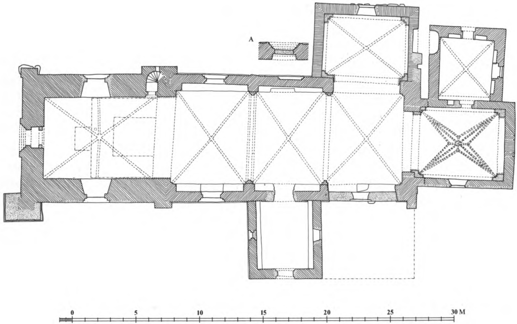
Fig.5. Plan. 1:300. A angiver skibets tilmurede norddør (s. 2566); på skibets sydside er med punkteret linie indtegnet den omtrentlige udstrækning af søndre \dagger korsarm (s. 2580). Målt af HeJ 1981, tegnet og suppleret af Mogens Vedsø 1991. Signaturforklaring s. 9. - Ground-plan. a. denotes the nave's walled up north door. The approximate extent of the south \dagger transept is denoted by a stippled line on the south side of the nave. Key on p. 9.
