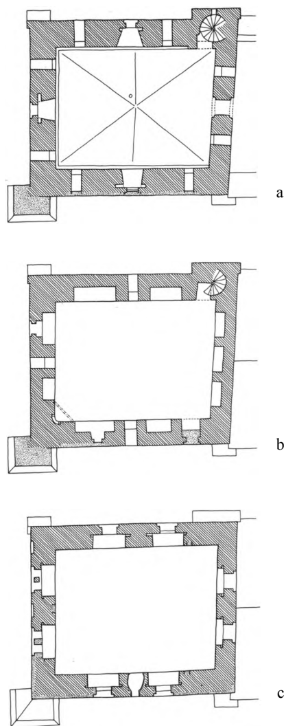
Fig. 6a-c. Planer. 1:300. Tårnets øvre stokværk. a. 1. mellemstokværk. b. 2. mellemstokværk. c. Klokkestokværket. Målt og tegnet af Mogens Vedsø 1989 og 1991. -a-c. Plans. Upper storeys of the tower. a. 1. middle storey. b. 2. middle storey. c. Belfry storey.
