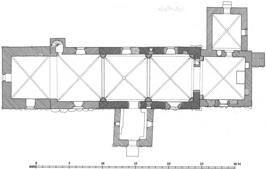
Fig.4. Plan. 1:300. Målt af HeJ 1981, suppleret og tegnet af Mogens Vedsø 1989 og 1991. Signaturforklaring s. 9. - Ground-plan. Key on p. 9.
