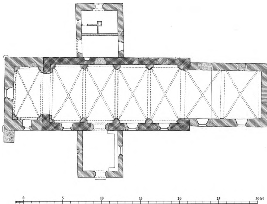
Fig.4. Plan. 1:300. Målt af HeJ 1981, suppleret og tegnet af Mogens Vedsø 1991. Signaturforklaring s. 9. - Ground-plan. Key on p. 9.
