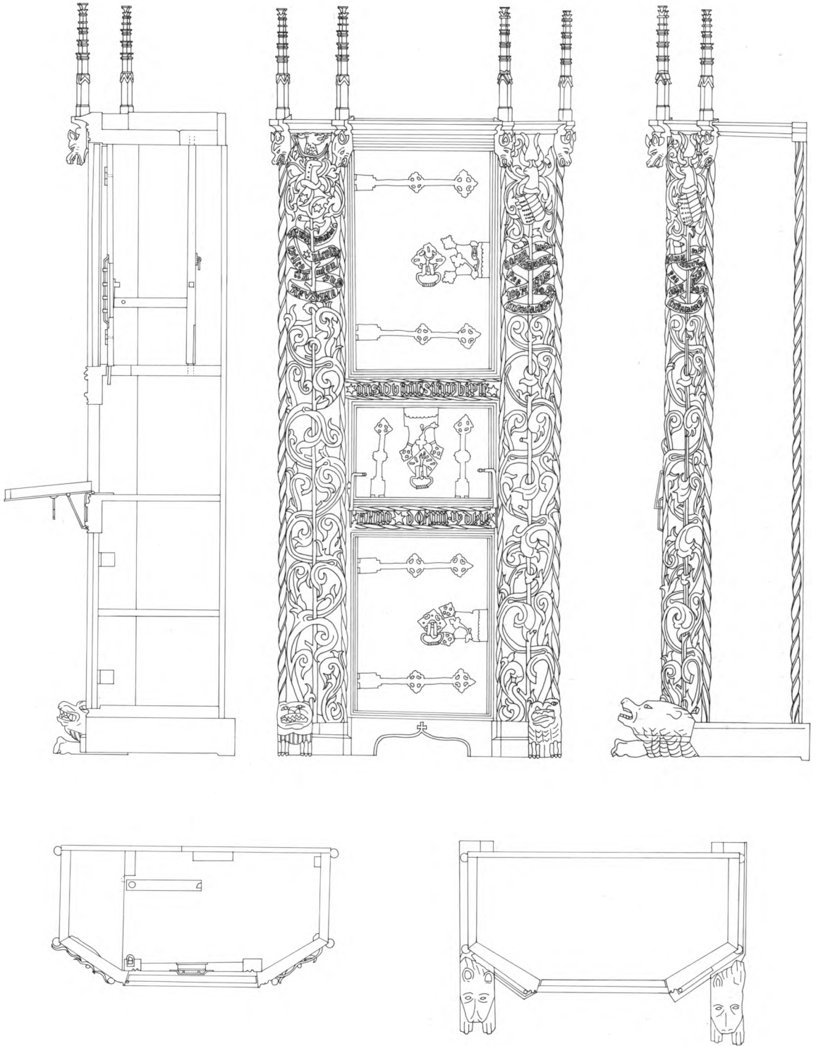
Fig.45. Monstransskab med skåret årstal 1519, opmåling ved John Bennetzen 1991. 1: 20 (s. 2783). - Cupboard with the carved date 1519.
