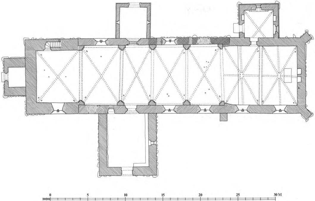
Fig.5. Plan. 1:300. Målt af HeJ 1981, tegnet af Mogens Vedsø 1991. Signaturforklaring s. 9. - Ground-plan. Key on p. 9.
