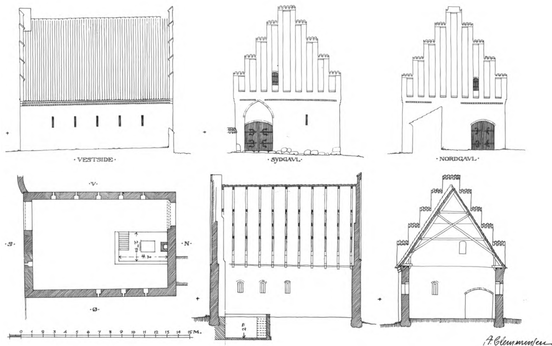
Fig. 26. Kirkelade (s. 3034). Plan, snit og facader 1:300. Forslag til istandsættelse ved Andreas Clemmensen 1917-18. - Tithe barn. Plan, sections and facades. Proposal for restoration submitted by Andreas Clemmensen, 1917-18.
