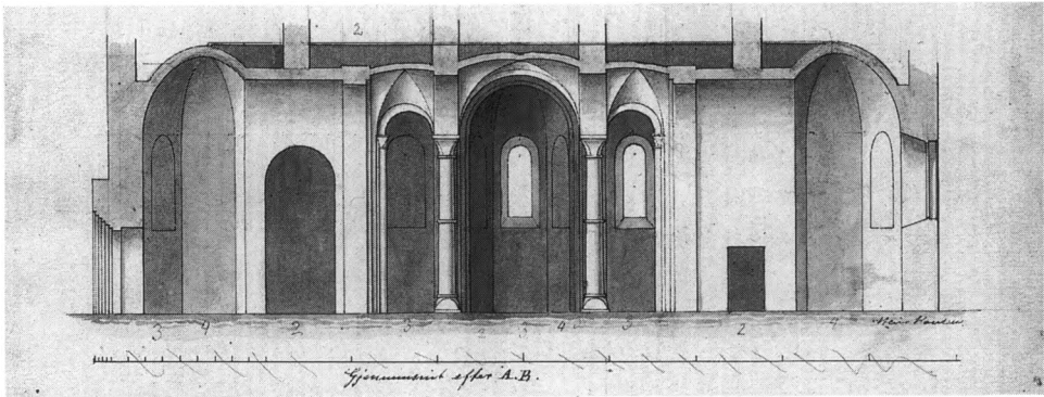
Fig. 43. Snit efter nord-sydaksen, set mod øst og med angivelse af skibets \dagger støtte- og hvælvsystem. 1:300. Målt og tegnet af Heinrich Hansen 1859. - Section of the north-south axis looking east and showing the nave's \dagger support and vault system.
