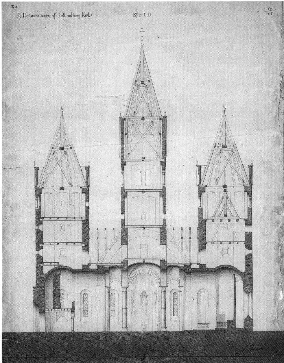
Fig. 116. Snit efter øst-vestaksen, set mod nord. 1:300. Restaureringsprojekt ved Vilhelm Tvede 1863. - Section of the east-west axis looking north. Restoration project by Vilhelm Tvede, 1863.
