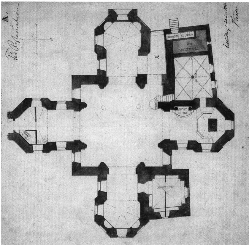
Fig. 42. Plan. 1:300. Målt og tegnet af Vilhelm Tvede, februar 1857. - Plan measured and drawn by Vilhelm Tvede, 1857.
