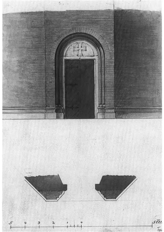
Fig. 122. Udkast til vestportal (s. 3127). 1:100. Udateret tegning ved Vilhelm Tvede. - Proposal for the west portal.
