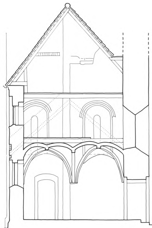
Fig. 102. Tværsnit af sakristiet, set mod syd. Tagspor efter to lavere \uparrow bygninger ses på kirkens østre korsarm, jfr. fig. 104 (s. 3100). 1:100. Målt af John Bennetzen 1992, tegnet af MN 1995. - Cross section of the sacristy looking south. Roof traces from two lower \uparrow buildings can be discerned on the east transept of the church, cf fig. 104.
