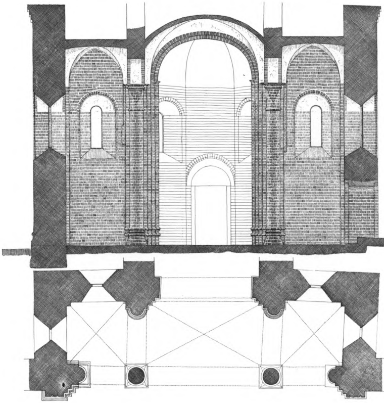
Fig. 52. Snit i skibets nordfag, set mod nord. 1:150. Målt og tegnet af Mogens Clemmensen 1921. - Section of the nave's north bay looking north.
