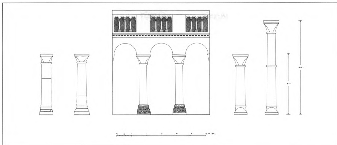
Fig. 100. Søjlestudier, som demonstrerer dimensionerne af en række granit søjler i sjællandske kirker (s. 3097). Fra venstre: Roskilde domkirkes koromgang, Helligtrekongers kapel smst., vestpulpitur i Fjenneslev samt Kalundborg, Vor Frue (uden og med øvre skafled). 1:150. Tegnet af C. M. Smidt. - Studies of pillars demonstrating the dimensions of a number of granite pillars in Zealand churches. From the left: Roskilde Cathedral's ambulatory, the Cathedral's Chapel of the Three Magi, the west gallery in the church of Fjenneslev, and Our Lady, Kalundborg (with and without the upper shaft).
