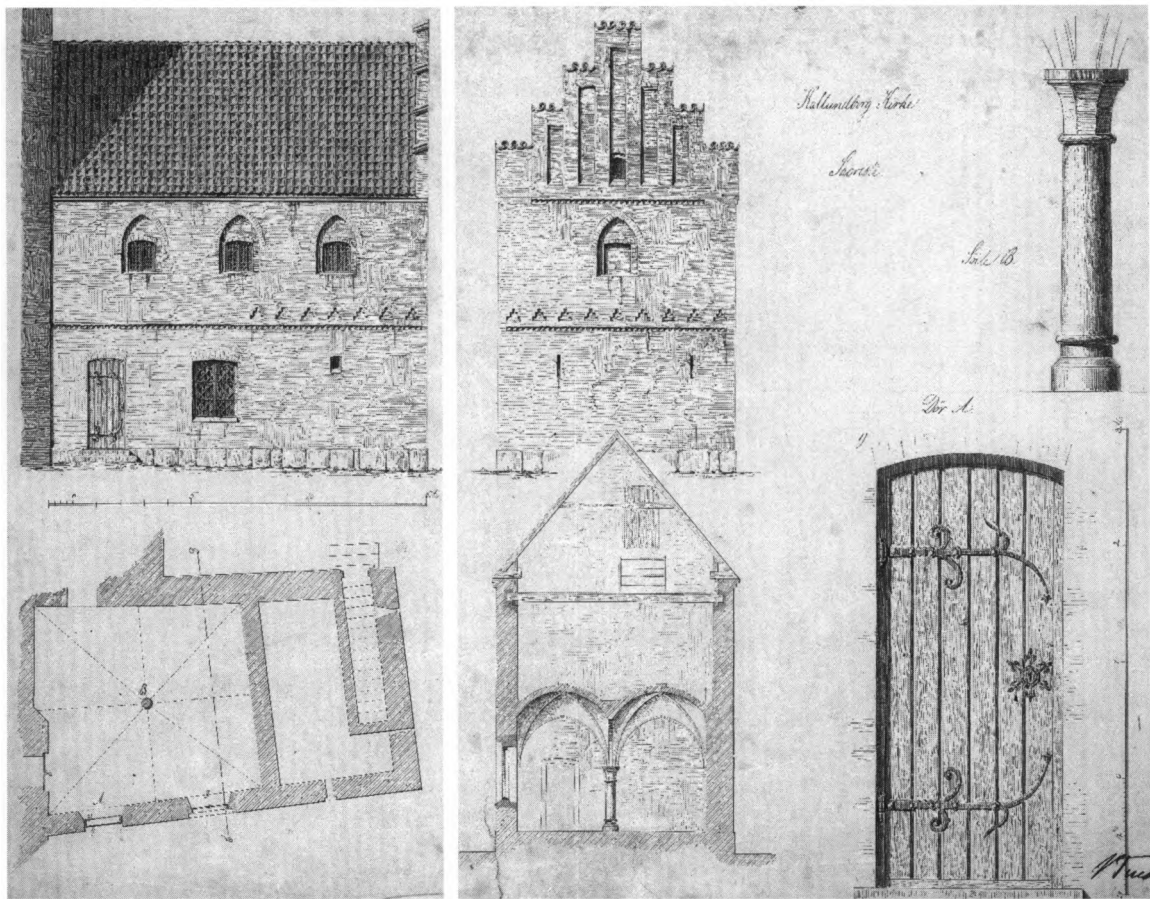
Fig. 101. Plan, snit, facader og detaljer af sakristi (s. 3100). Hovedtegningerne 1:200. Restaureringsprojekt ved Vilhelm Tvede 1871. - Plan, sections, facades and details of the sacristy. Restoration project by Vilhelm Tvede, 1871.
