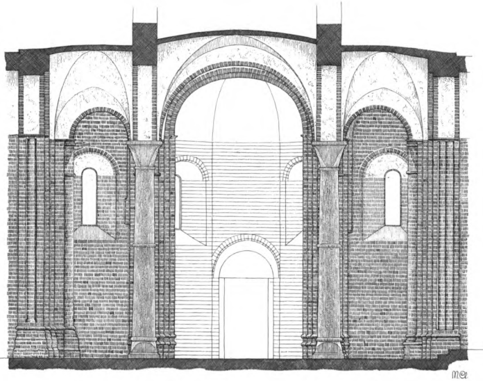
Fig. 53. Snit i skibet efter øst-vestaksen, set mod nord. 1:150. Målt og tegnet af Mogens Clemmensen 1921. - Section of nave on east-west axis looking north.
