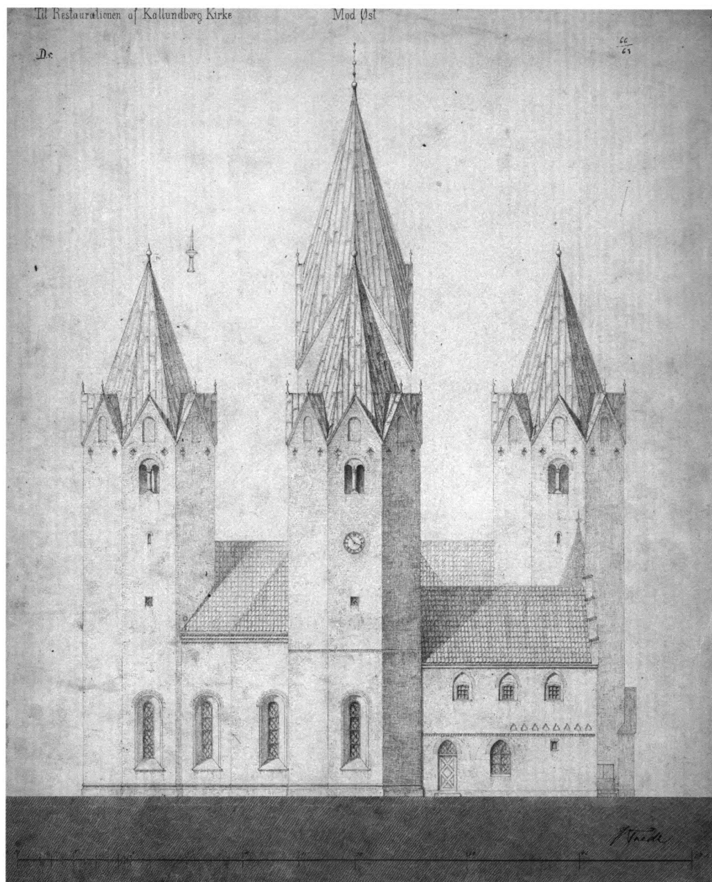
Fig. 117. Facade mod øst. 1:300. Restaureringsprojekt ved Vilhelm Tvede 1863. - East facade. Restoration project by Vilhelm Tvede, 1863.
