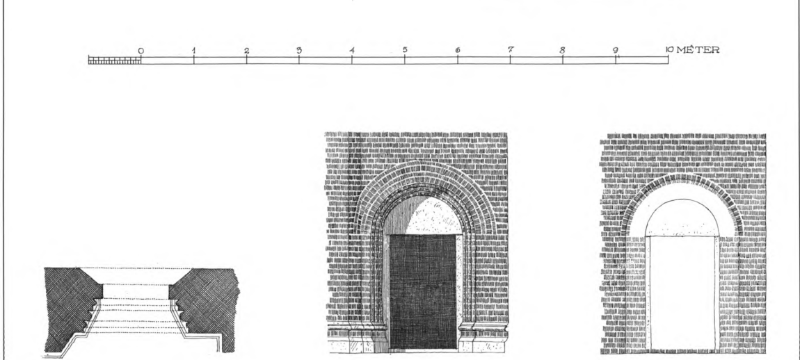
Fig. 56. Plan og facader af østportal (s. 3072). 1:100. Målt og tegnet af Frederik Jensen o. 1921. - Plan and facades of the east portal.
