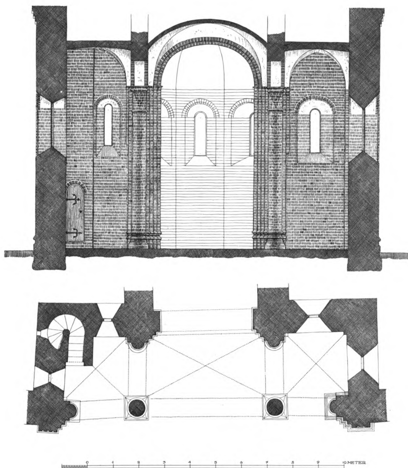
Fig. 51. Snit i skibets sydfag, set mod syd. 1:150. Målt og tegnet af Mogens Clemmensen 1921. - Section of the nave's south bay looking south.
