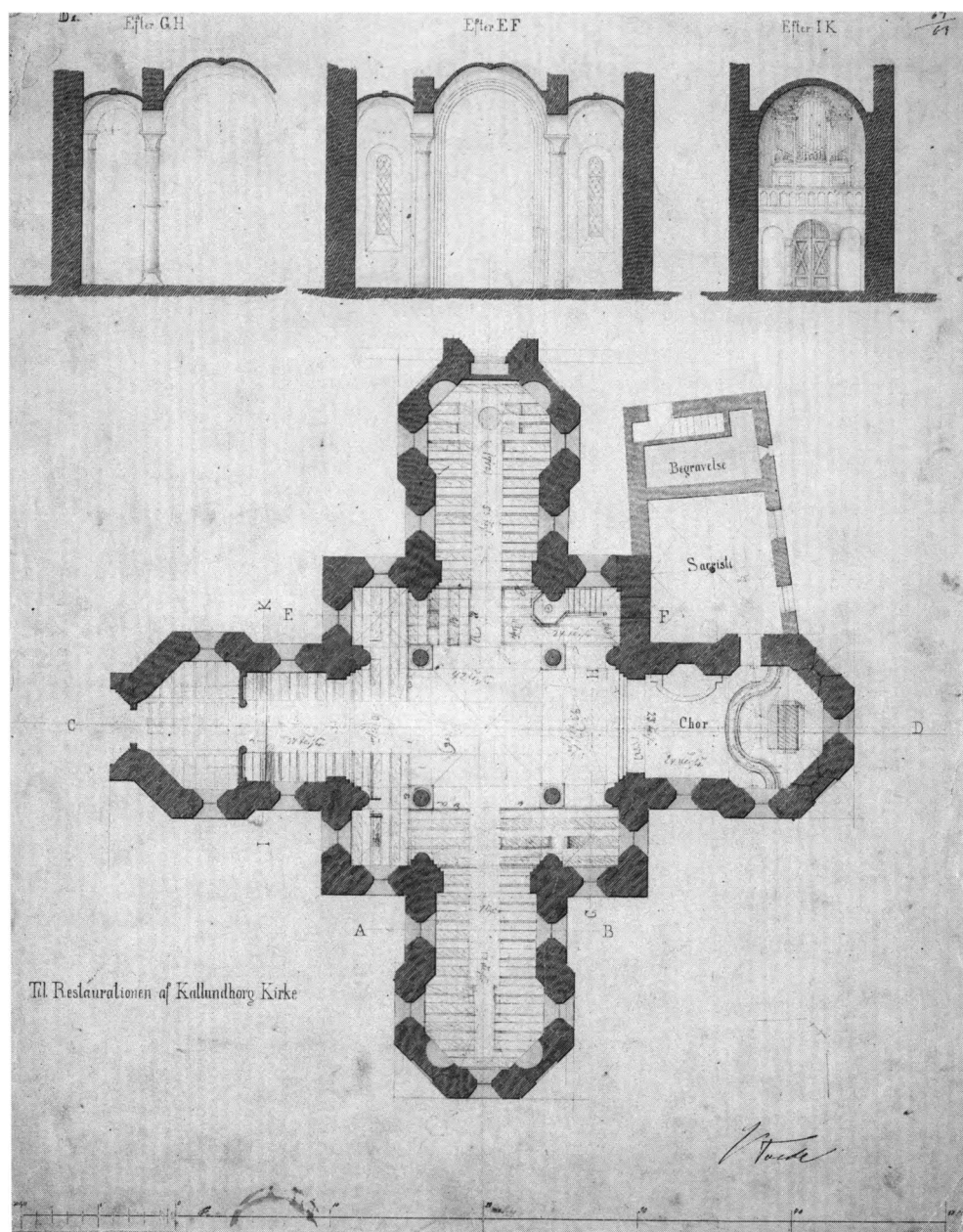
Fig. 115. Plan og snit. 1:300. Restaureringsprojekt ved Vilhelm Tvede 1863. - Plan and section. Restoration project by Vilhelm Tvede, 1863.
