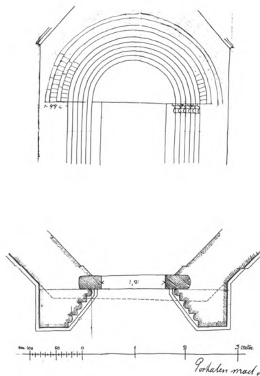
Fig. 71. Forslag til nordportal (s. 3078). 1:100. Mogens Clemmensen 1918. Kunsthøgskolens Bibliotek. - Proposal for the north portal.
