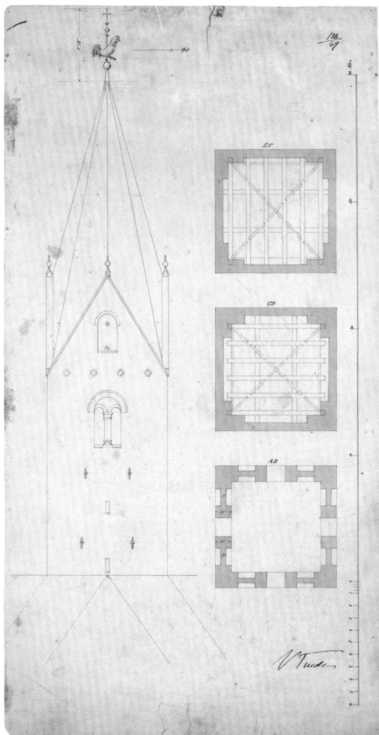
Fig. 120. Etageplaner og facade af midtertårn. 1:200. Restaureringsprojekt ved Vilhelm Tvede 1869. - Storey plans and facade of the central tower. Restoration project by Vilhelm Tvede, 1869.
