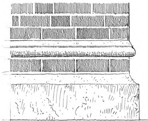
Fig. 64. Sokkel (s. 3070). 1:20. Målt og tegnet af Mogens Clemmensen 1921. - Base.
