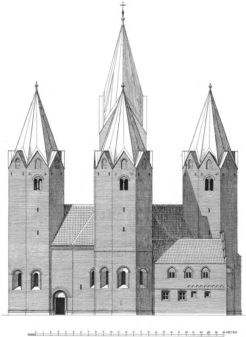
Fig. 50. Facade mod øst. 1:300. Målt og tegnet af Frederik Jensen o. 1921. - East facade.
