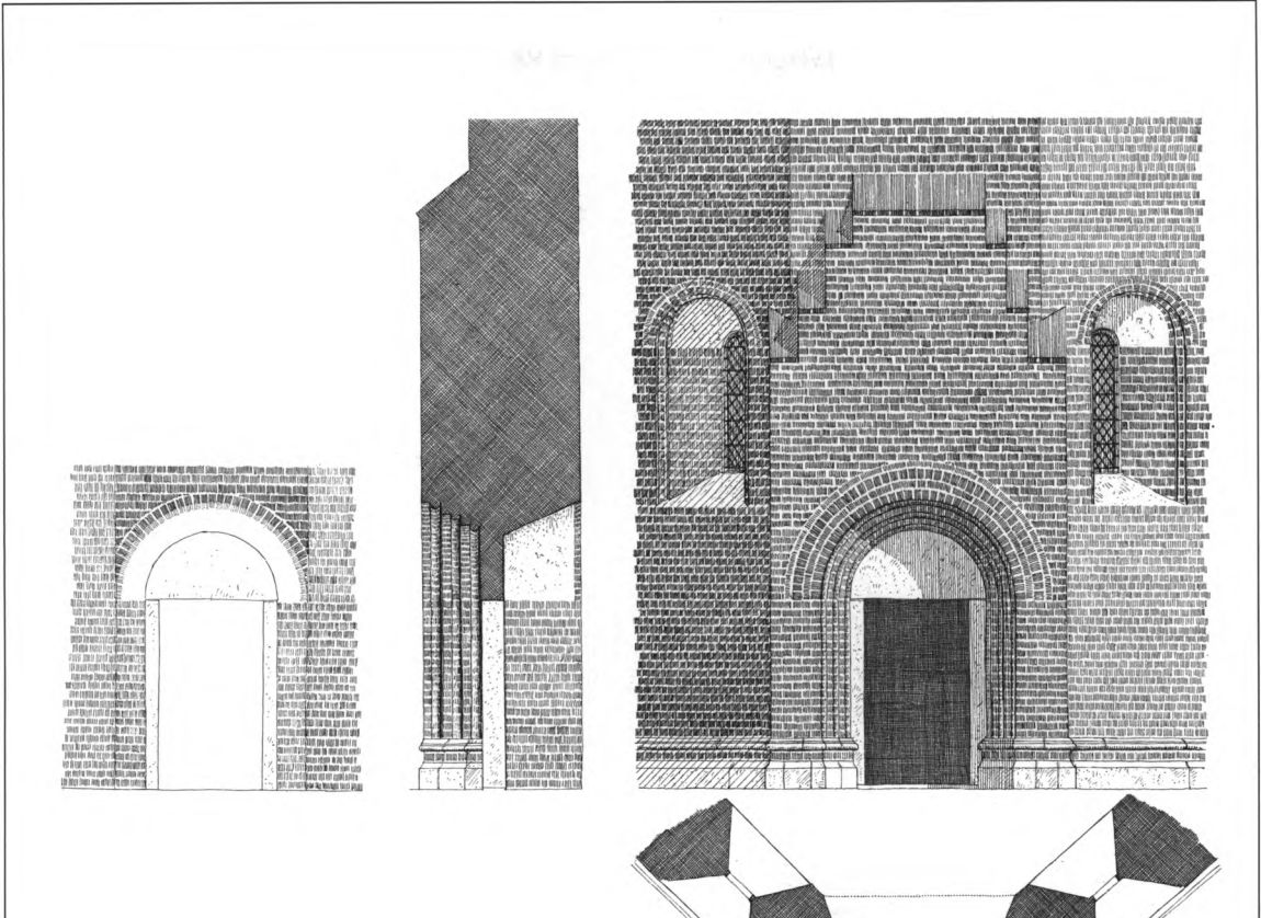
Fig. 55. Plan, facade og snit af nordportal (s. 3077). 1:100. Målt og tegnet af Frederik Jensen o. 1921. - Plan, façade and section of the north portal.
