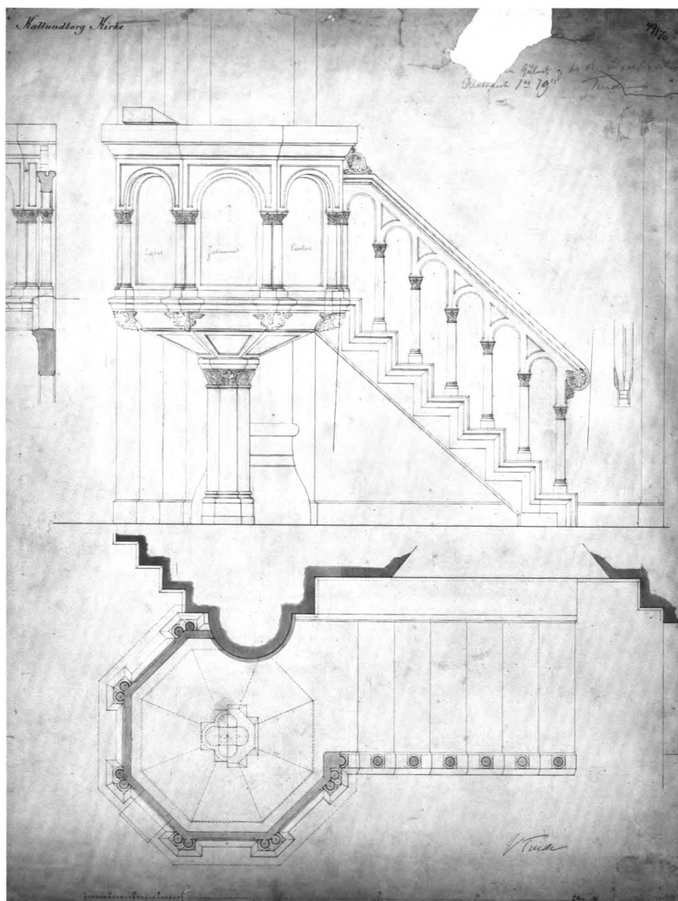
Fig. 162. Tegning af Vilhelm Tvede 1871 til prædikestolen, sml. fig. 136 og 163 (s. 3163). I NM2. - Proposal for the pulpit drawn by Vilhelm Tvede in 1871, cf. figs. 136 and 163.
