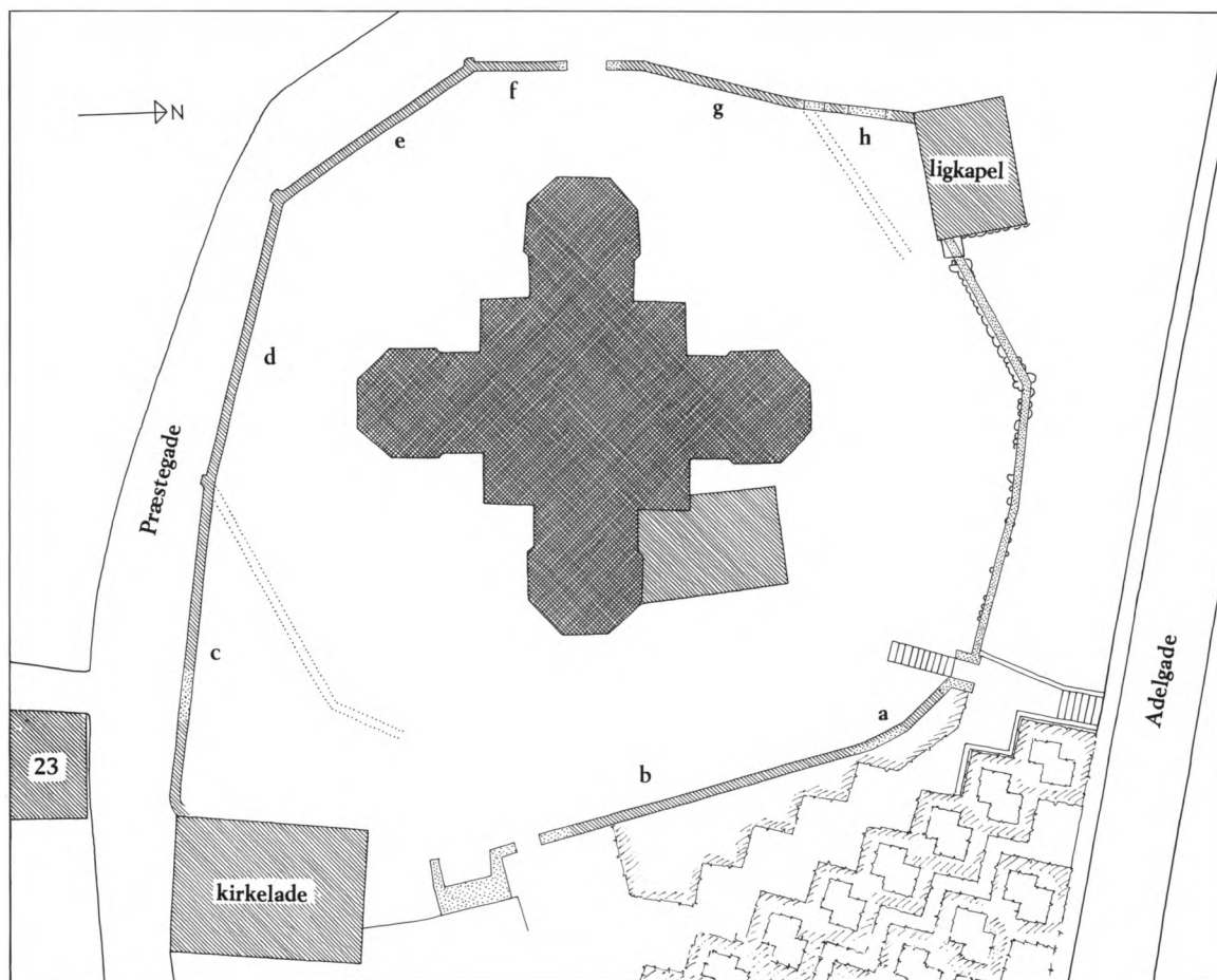
Fig. 11. Skitseplan af kirkegården med dens nærmeste omgivelser. Stiplede linjer angiver formodede ældre \dagger kirkegårdsmure (s. 3027). 1:500. Tegnet af MN 1995, bl.a. på grundlag af planer ved Marinus Andersen. - Sketch plan of the churchyard with its nearest surroundings. Dotted lines indicate presumed former \dagger churchyard walls.
