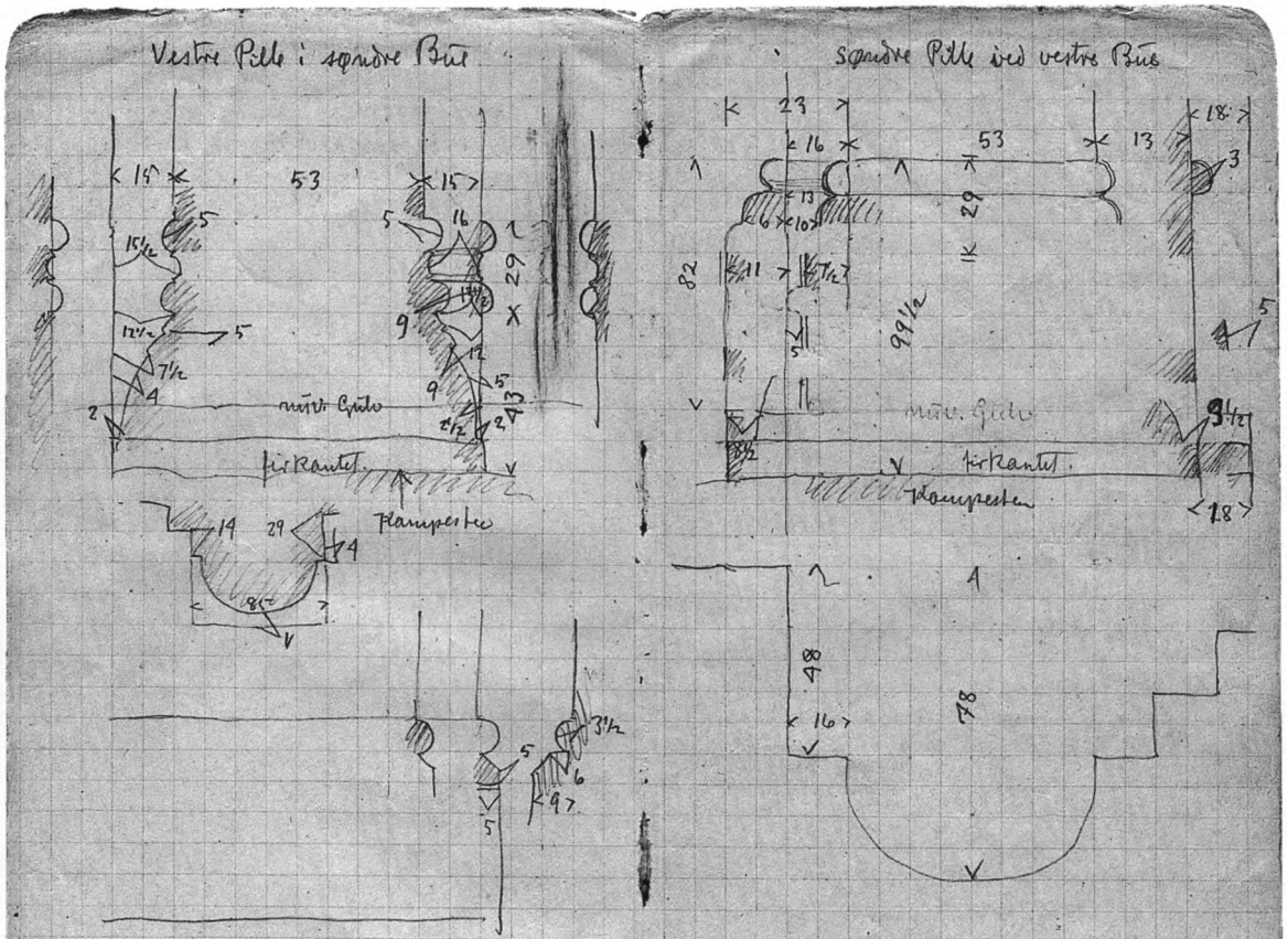
Fig. 233. Skitse o. 1920 af halvøjlebasen ved søndre og vestre korsarmsarkade, jfr. fig. 93 og 95 (s. 3092f.). Mogens Clemmensens notebog IV. - Sketches c. 1920 of bases of engaged columns by the arcades of the south and west transepts, cf. figs. 93 and 95.
