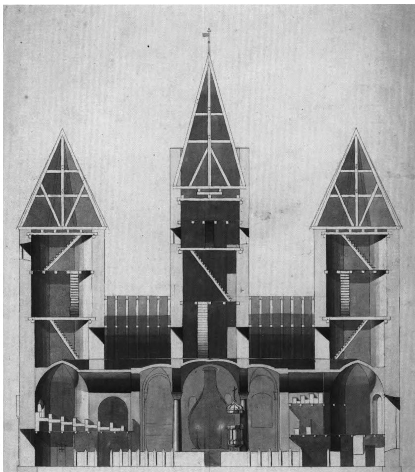
Fig. 38. Snit nord-syd. 1:300. Formentlig målt og tegnet af C. B. Hornbech o. 1820. - North-south section Probably measured and drawn by C. B. Hornbech, c. 1820.
