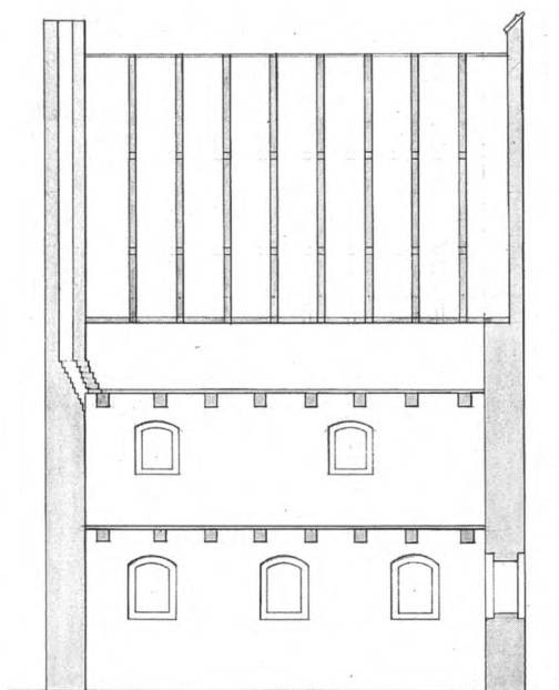
Fig. 28a-e. »Rektorboligen«, nu ligkapel (s. 3039). a. Facade mod syd. b. Planer i stue og overetage. c. Facade mod øst. d. Facade mod nord. e. Længdesnit mod nord. 1:150. Målt og tegnet af Jacob Kornerup og Vilhelm Tvede 1877. - »The Rector's house«, now the mortuary. a. South facade, b. Plans of ground floor and upper storey. c. East facade, d. North facade, e. Longitudinal section to the north. Measured and drawn by Jacob Kornerup and Vilhelm Tvede 1877.
