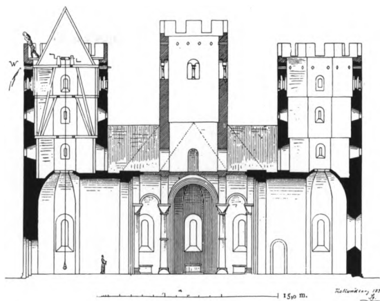
Fig. 34. Vor Frue som kirkeborg ifølge Seesselberg 1895 (s. 3047). Snit efter nord-sydaksen, set mod øst.
