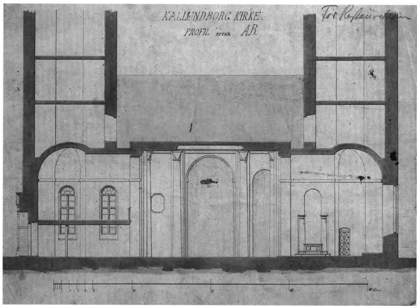
Fig. 41. Snit i øst-vestaksen, set mod nord. 1:300. Målt og tegnet af Vilhelm Tvede, februar 1857. - Section of east-west axis looking north. Measured and drawn by Vilhelm Tvede, 1857.
