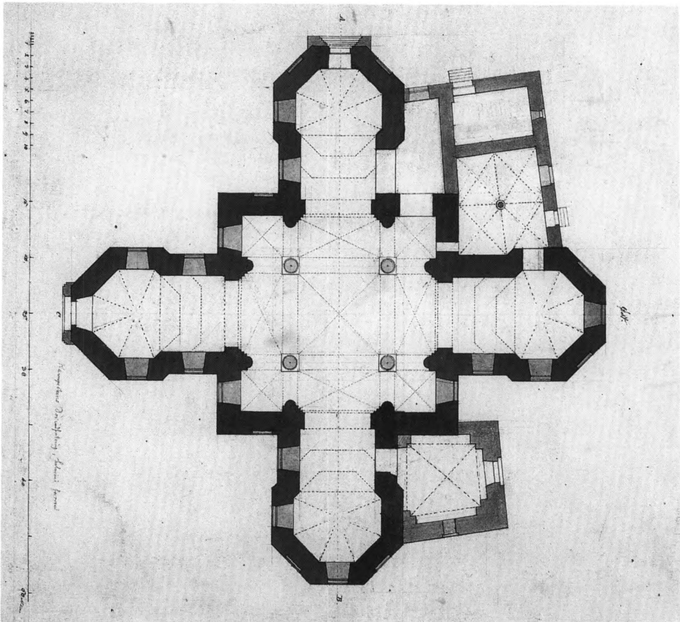
Fig. 44. Plan med angivelse af skibets \dagger støtte- og hvælvsystem. 1:300. Målt og tegnet af Heinrich Hansen 1859. - Plan showing the nave's \dagger support and vault system.
