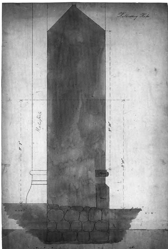
Fig. 62. Tværnsnit af skibets fundament og mur (s. 3068). 1:50. Udateret tegning ved Vilhelm Tvede. - Cross-section of the nave's foundation and wall.
