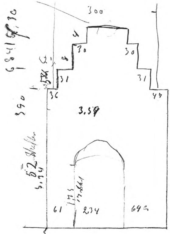
Fig. 230-31. Skitser til rekonstruktion af vest- og nordportal (s. 3076 og -78). Tegnet af murerformand Jørgensen o. 1920 i Mogens Clemmensens notebog VIII. - Sketch proposals for the reconstruction of the west and north portals.
