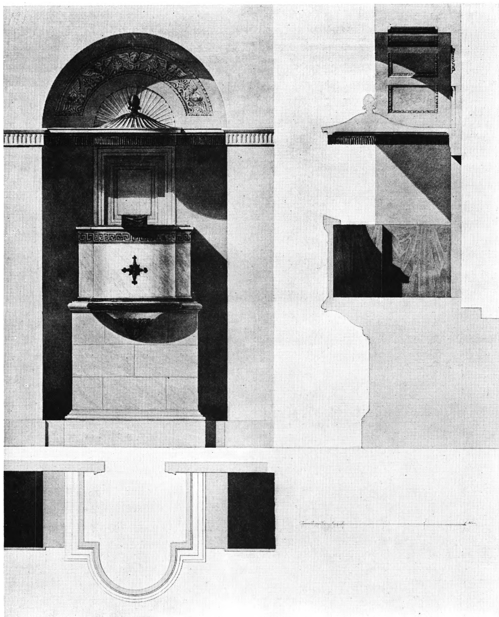
Fig. 115. Prædikestolen. Tegning af C. F. Hansen i Kirkens Arkiv.
