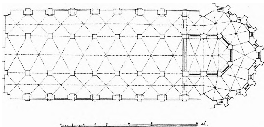
Fig. 7. Den gotiske Vor Frue Kirke. Efter J. F. Ramus' Projekt til Kirkens Genopførelse 1731 (sml. Bygningshistorie 1728—1807), idet Taarn og andre Tilbygninger er udeladt.
