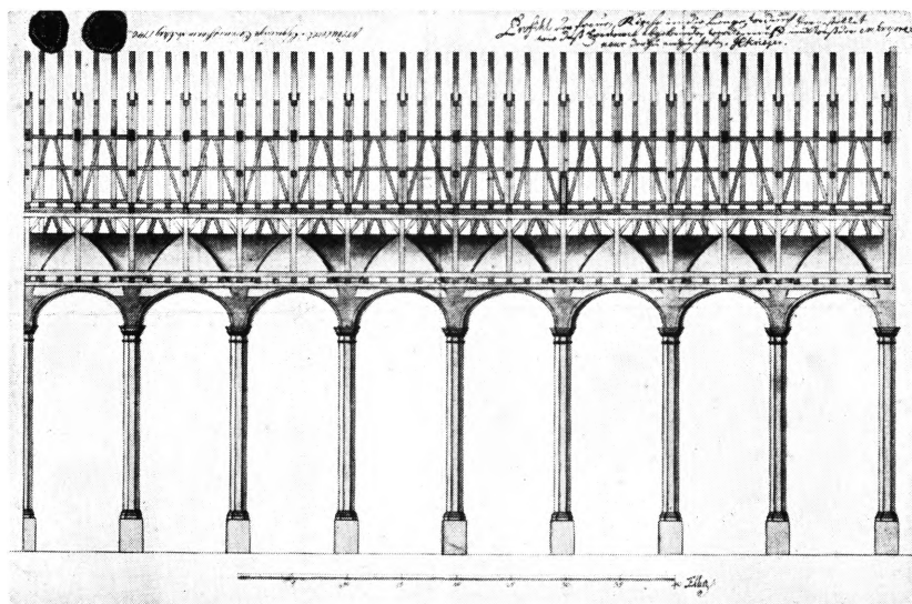
Fig. 66. Længdesnit i søndre Sideskib tegn et af J. G. Kreysig, paategnet af Krieger 1729 og forsynet med Lerches og Worms Segl.
