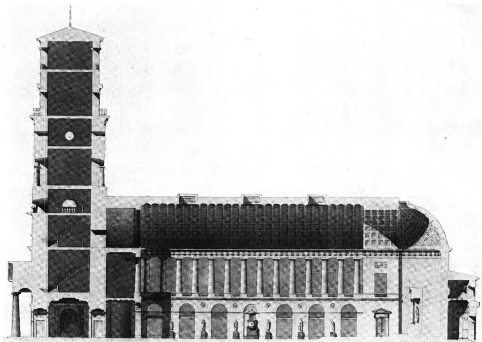
Fig. 98. Længdesnit i Kirken, efter G. F. Hetsch's Udgave af C. F. Hansens Bygninger 1847.
