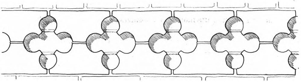
Fig. 14. Firkløverfrise 1:10. Rekonstrueret efter Formsten (Fig. 15,5).
