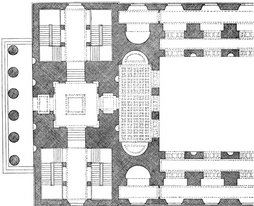
Fig. 104. Vor Frue Kirke. Planer 1:300. Øverst Pulpitur-Stokværk
