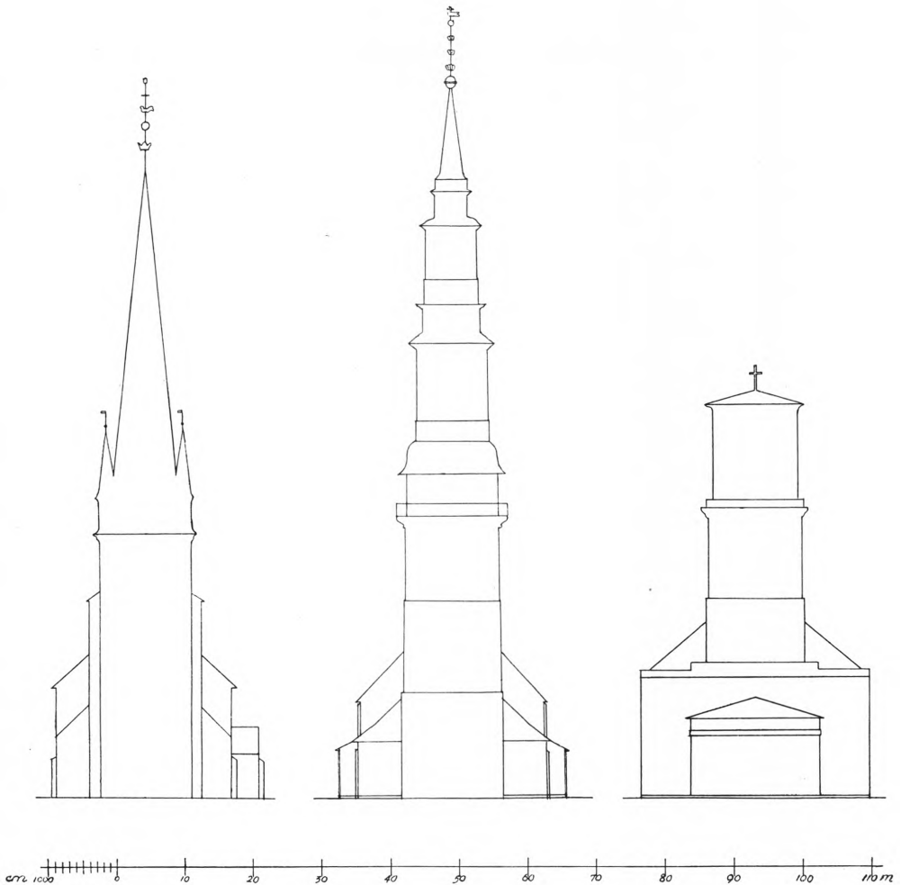
Fig. 22. Vor Frue Kirkes Taarne 1:1000.
