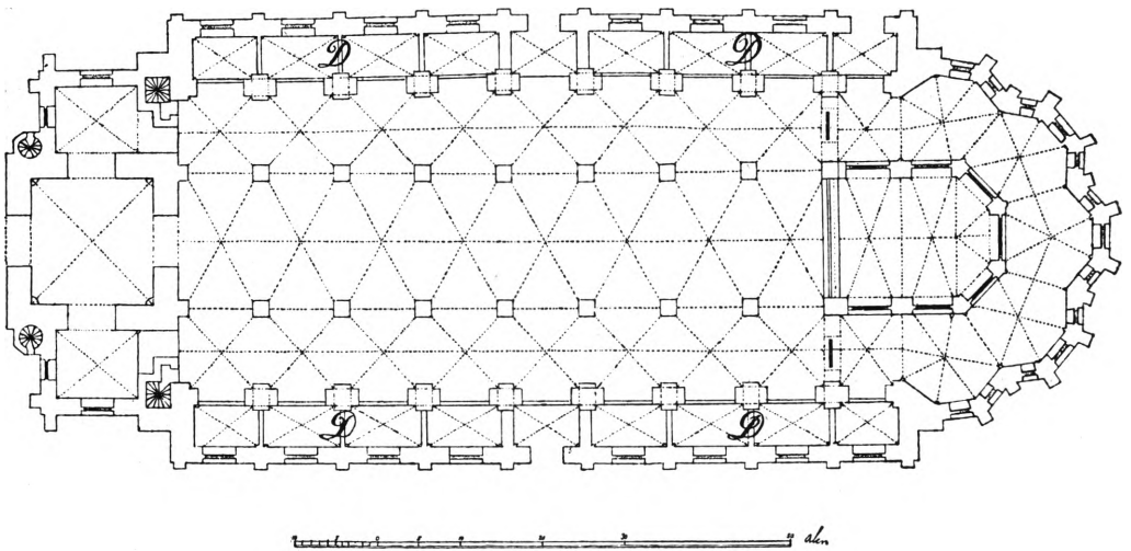
Fig. 69. J. F. Ramus' Plan fra 1731. Det middelalderlige Kor er bevaret, men Sydsidens Kapeller er erstattet af et ydre Sideskib, og et lignende er tilbygget paa Nordsiden D—D.
