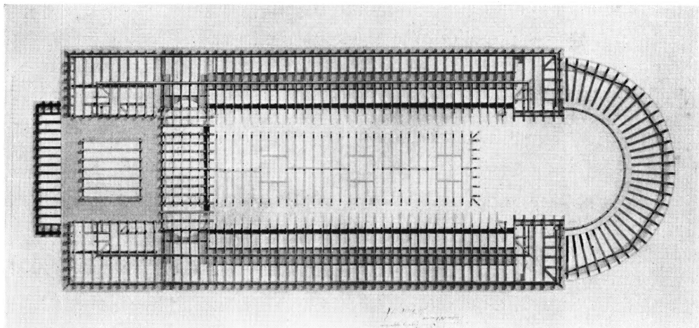
Fig. 95. Tagplan, dateret 1810, approberet 14. Juni 1811.
