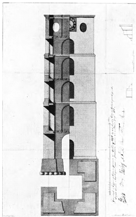
Fig. 76. Banner Matthiesens Arbejdstegning til Taarnet 1734.
