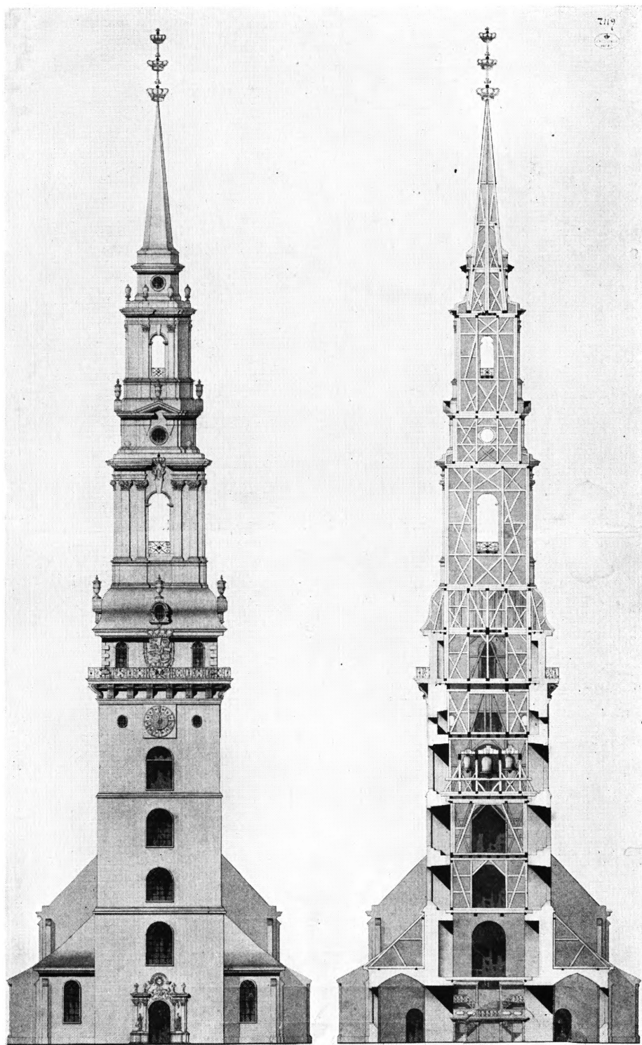
Fig. 84. Frue Kirkes Taarn, opmaalt af Tømremester, Major Wahl.
