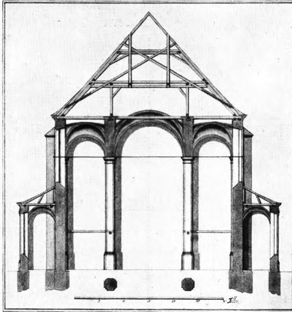
Fig. 68. Tværsnit af Skibet visende Hallekirken med firkantede Pilasterpiller og de ydre Sideskibe. Tegnet af J. G. Kreysig.
