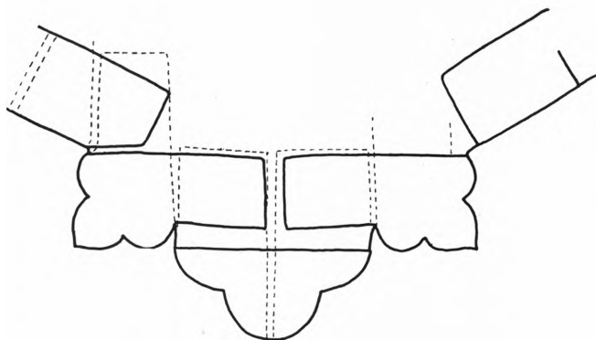
Fig. 12. Profil af Hjørnepille mod Kor-Omgangen, 1:10.
