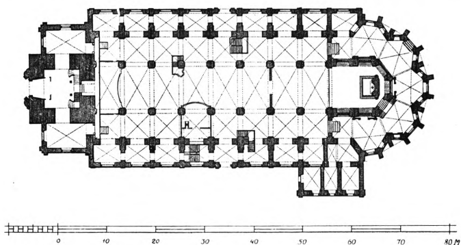
Fig. 79-80. Sydside og Plan af Vor Frue Kirke. Efter »Danske Vitruvius« 1746.
