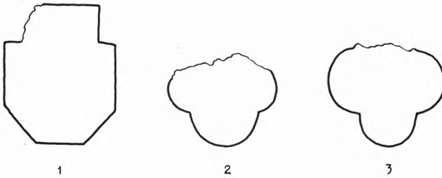
Fig. 6. Romanske Profilsten 1:10.
