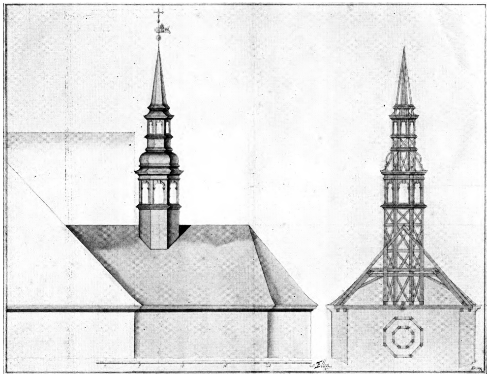
Fig. 81. Tagrytteren over Koret; tegnet af J. G. Kreysig.
