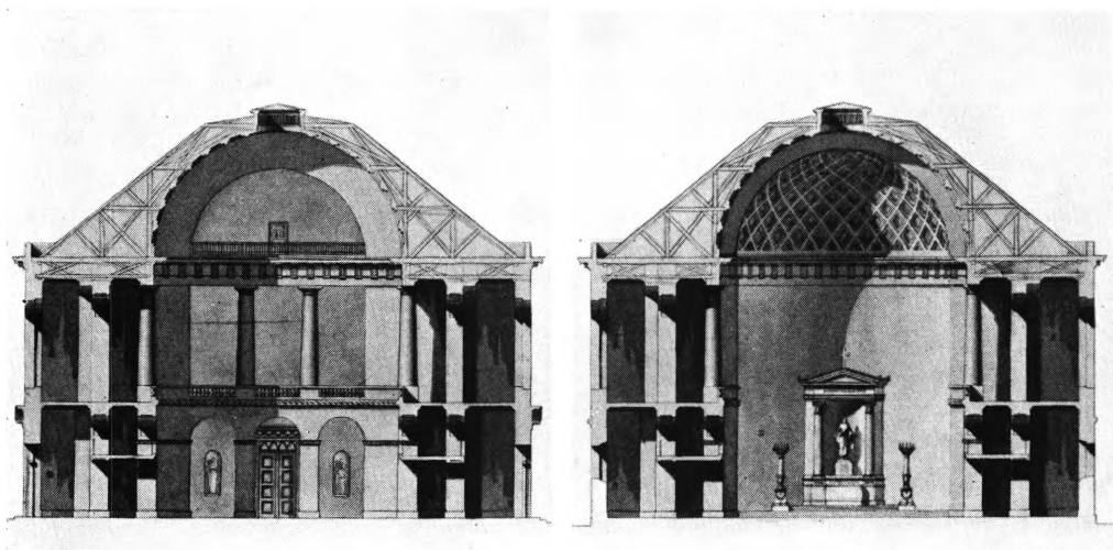
Fig. 99. Tværsnit i Skibet, efter G. F. Hetsch's Udgave af C. F. Hansens Bygninger 1847. Til venstre set mod Indgangen, til højre set mod Alteret.
