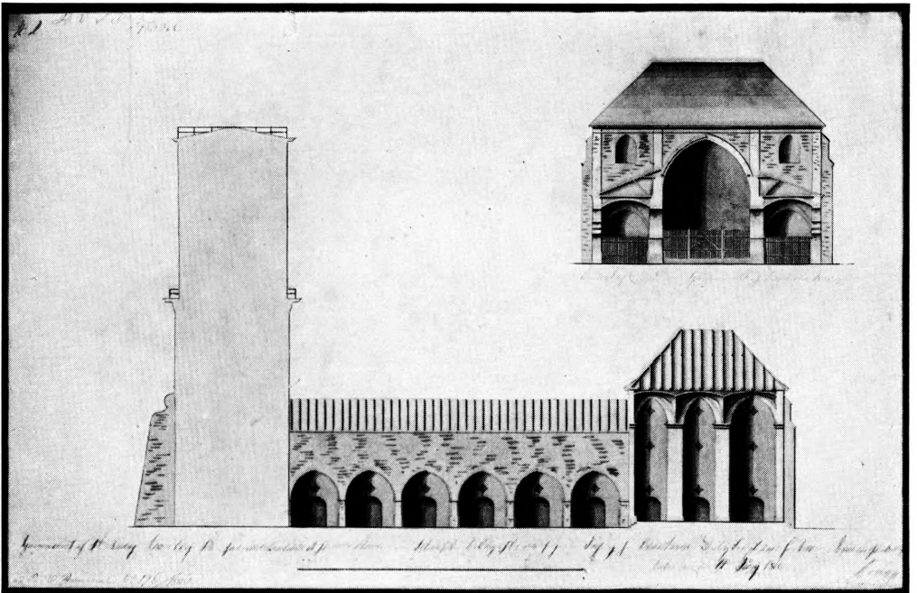
Fig. 42. S. Nicolai kirke. Snit af bygningen, omdannet til brandstation, tegnet af A. Kirkerup 1806. Stadsarkivet.
