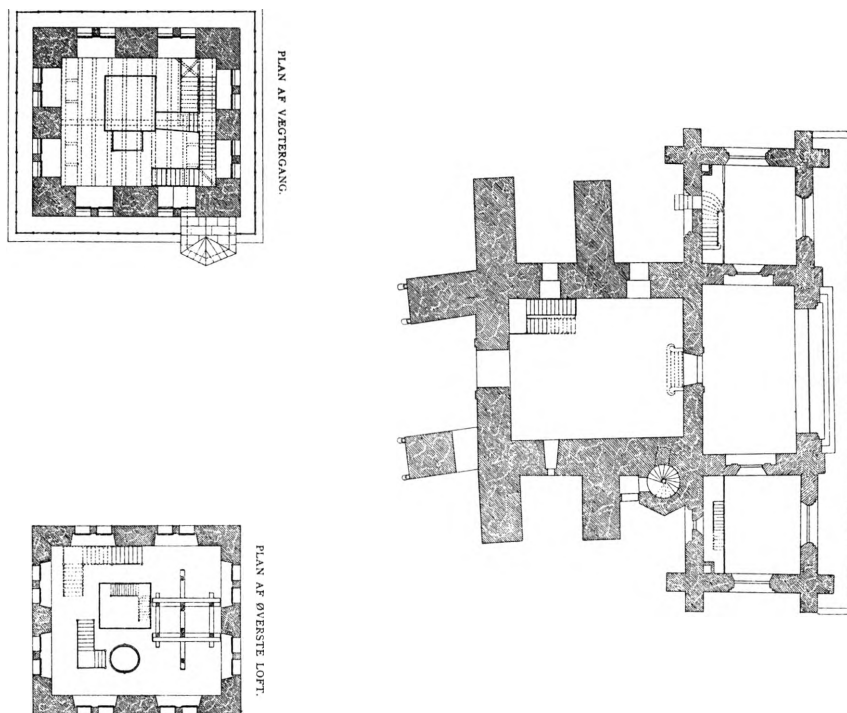
Fig. 17. S. Nicolai kirke. Planer af tre stokværk. Foreningen af 3. Dec.
