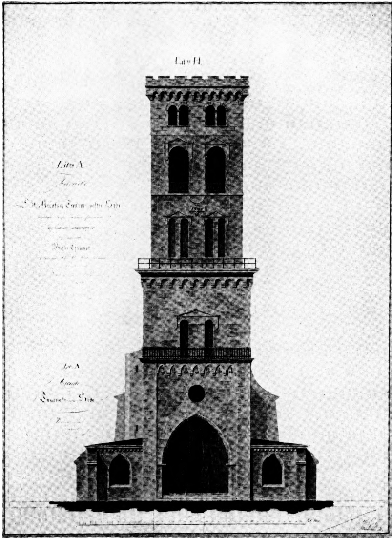
Fig. 48. S. Nicolai kirke. H. C. Schmidts endelige udkast til Nicolai tårns øvre afslutning 1820, tilføjet med en klap på udkastet fra 1816.
