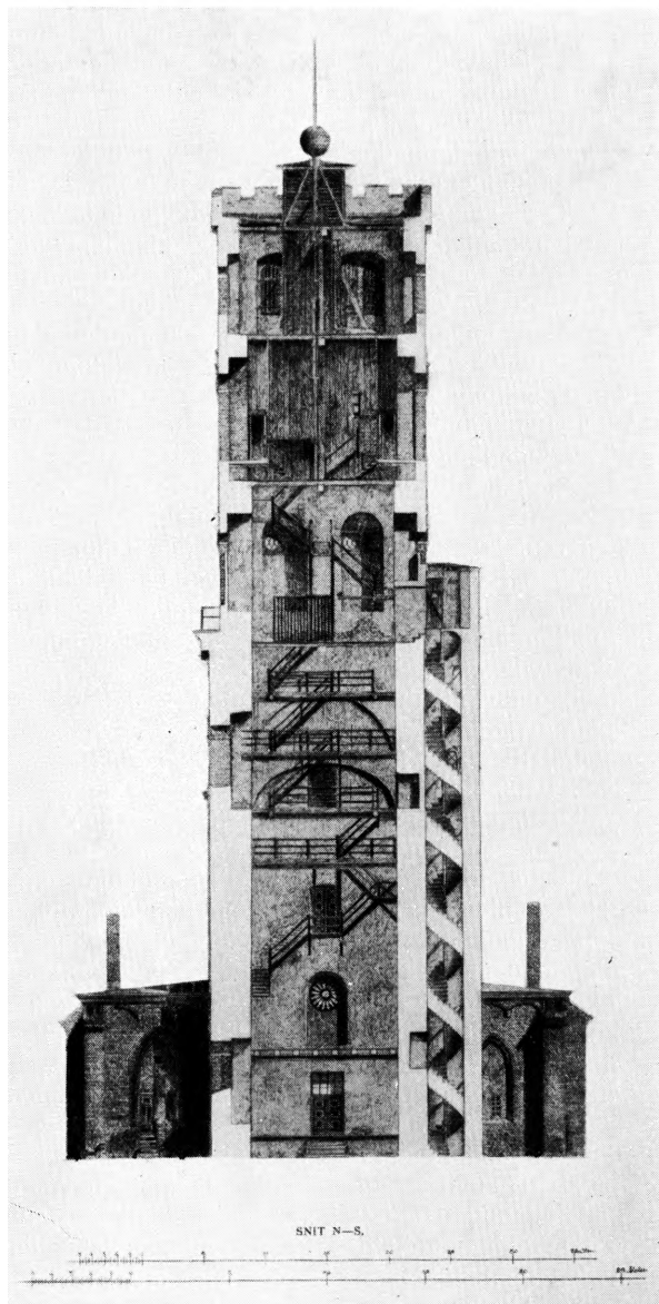
Eig. 19. S. Nicolai kirke. Snit af tårnet nord-syd. Foreningen af 3. Dec.
