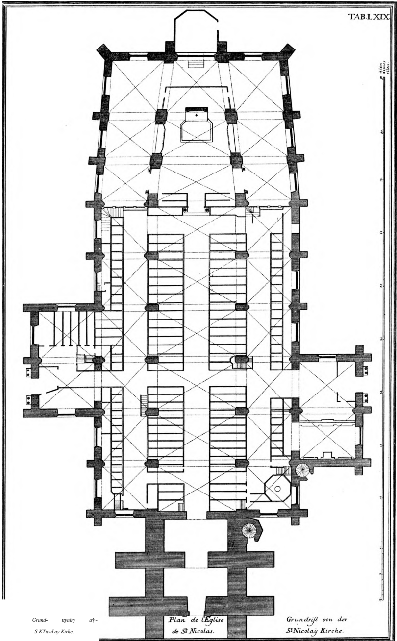
Fig. 10. S. Nicolai kirkes grundplan. Efter Danske Vitruvius.
