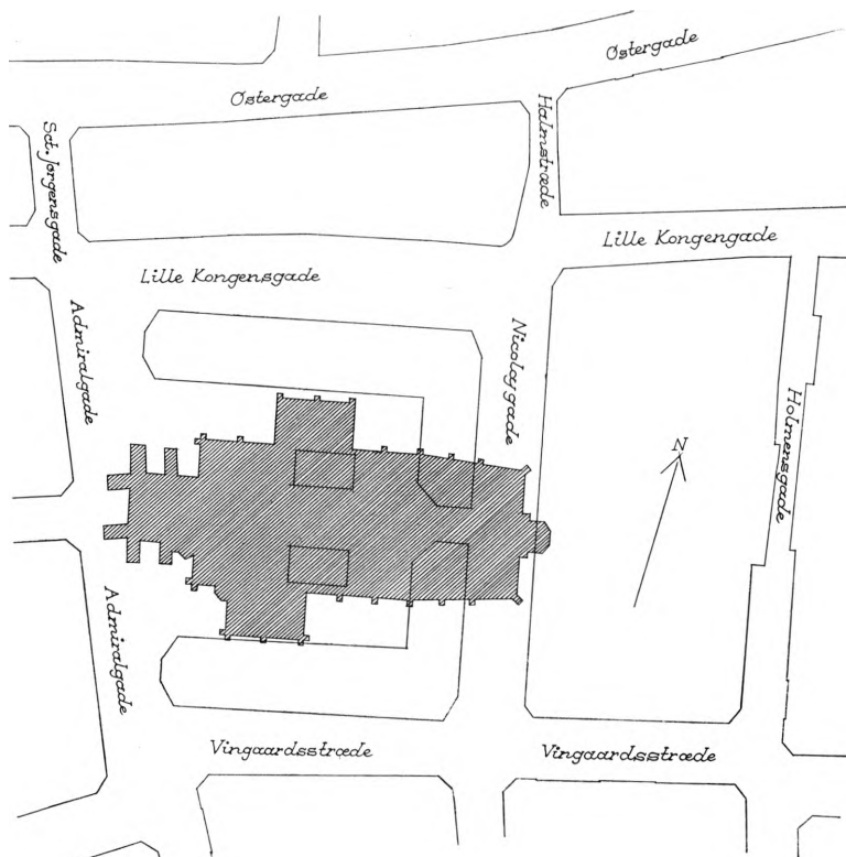
Fig. 5. S. Nicolai. Kirkens plan efter Danske Vitruvius indtegnet i det moderne gadenet af Jørgen Holck-Christiansen.
