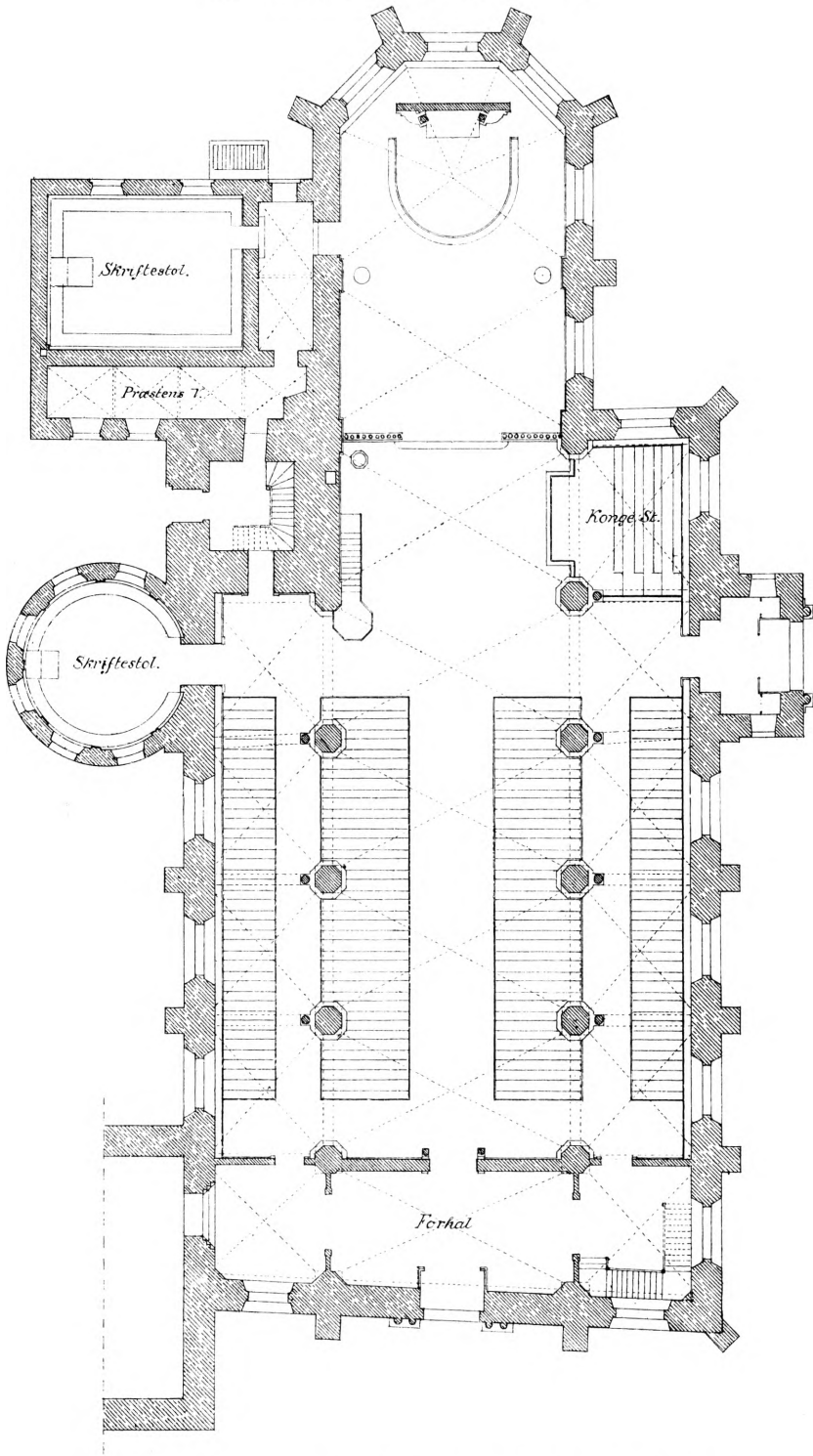
Fig. 23. Helligåndskirken. Plan, 1:300. Målt af H. Storck 1878. Øst opad.
