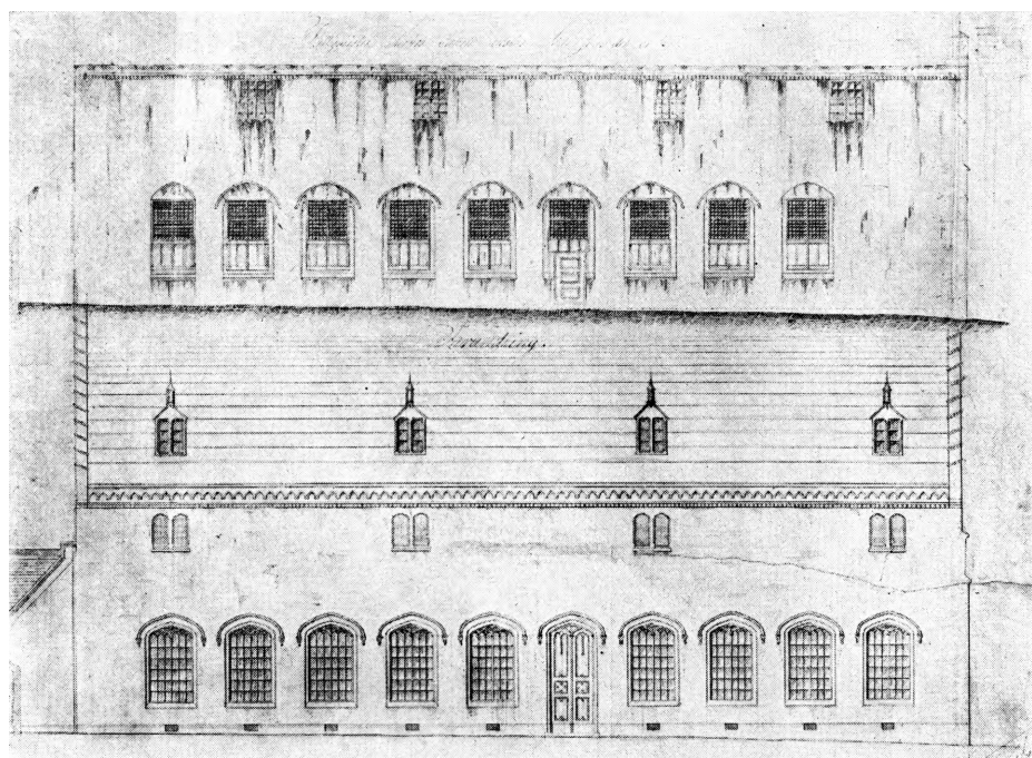
Fig. 13. Helligåndshuset. Façade og vestvæg. Tegning af P. Chr. Kramp 1846.
