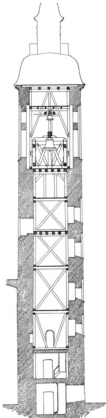
Fig. 16. Helligåndskirkens tårn. Snit 1878 af H. Storek.
