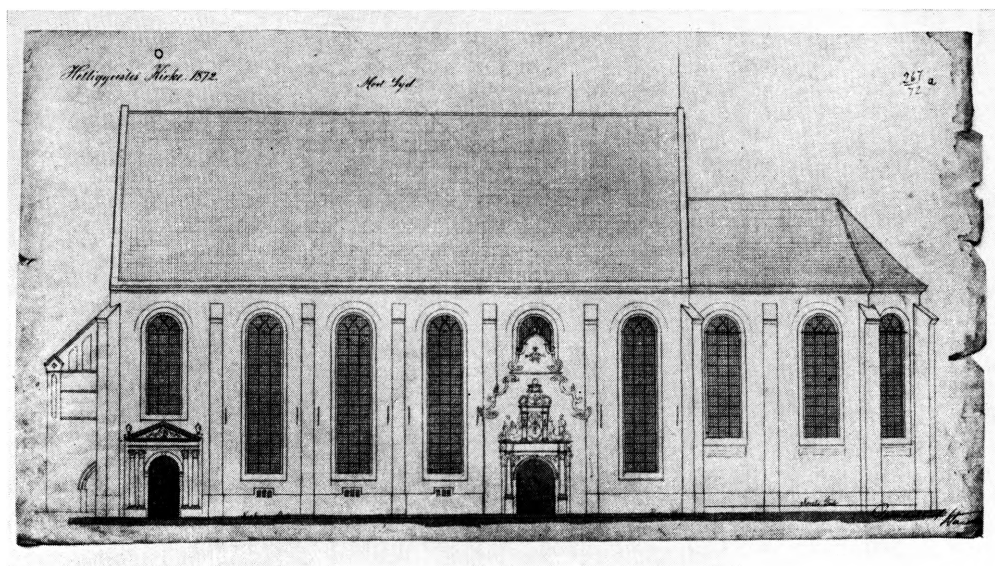
Fig. 20. Helligåndskirkens sydfaçade. Målt 1872 af V. Tvede.
