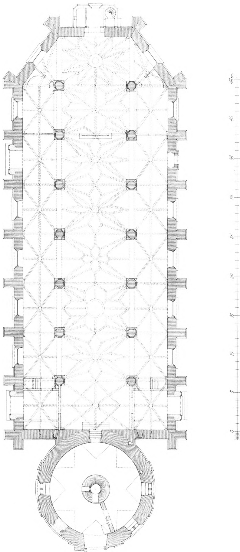
Fig. 12. Trinitatis kirke. Plan 1:300. Opmålt 1923—25 af Helge Finsen og Flemming Teisen. Eftertegnet 1961 af Holger Schmidt.
