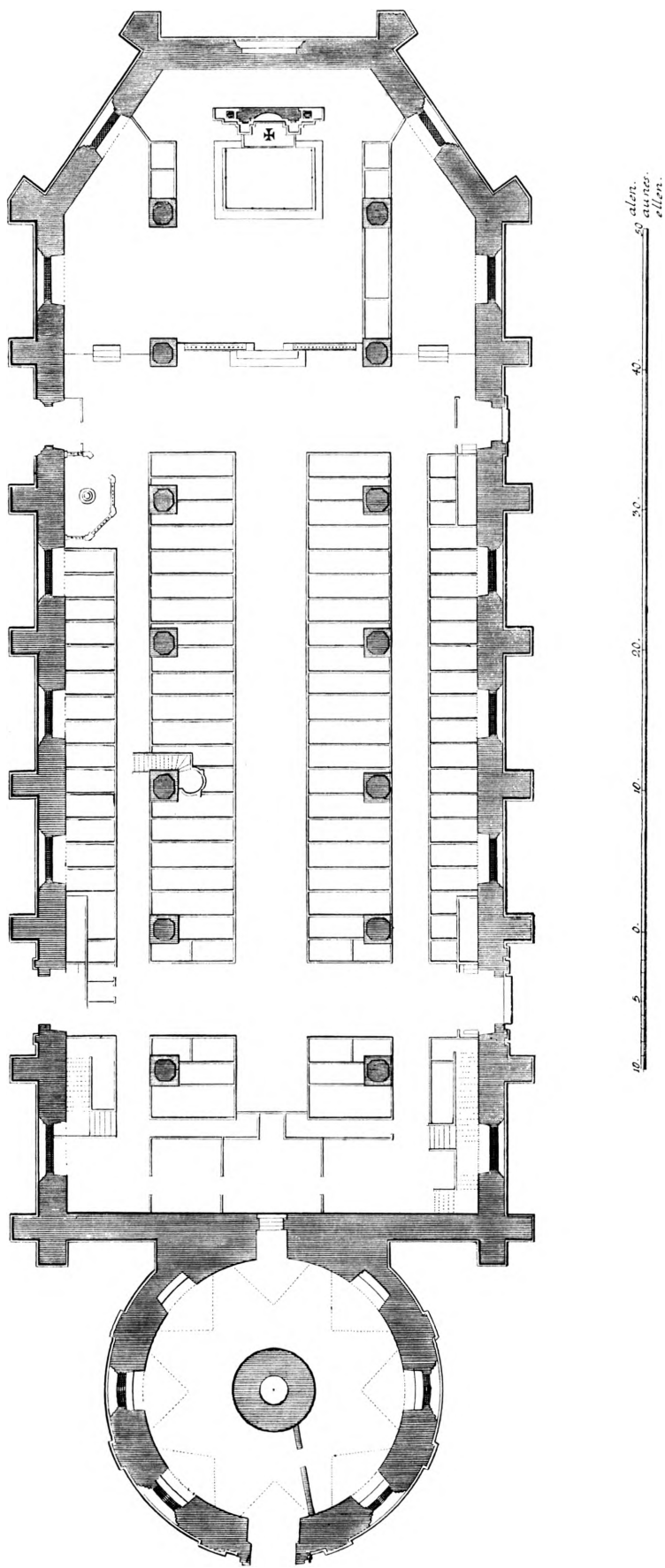
Fig. 13. Trinitatis kirke. Plan 1:300. Efter Thurahs Danske Vitruvius 1746.
