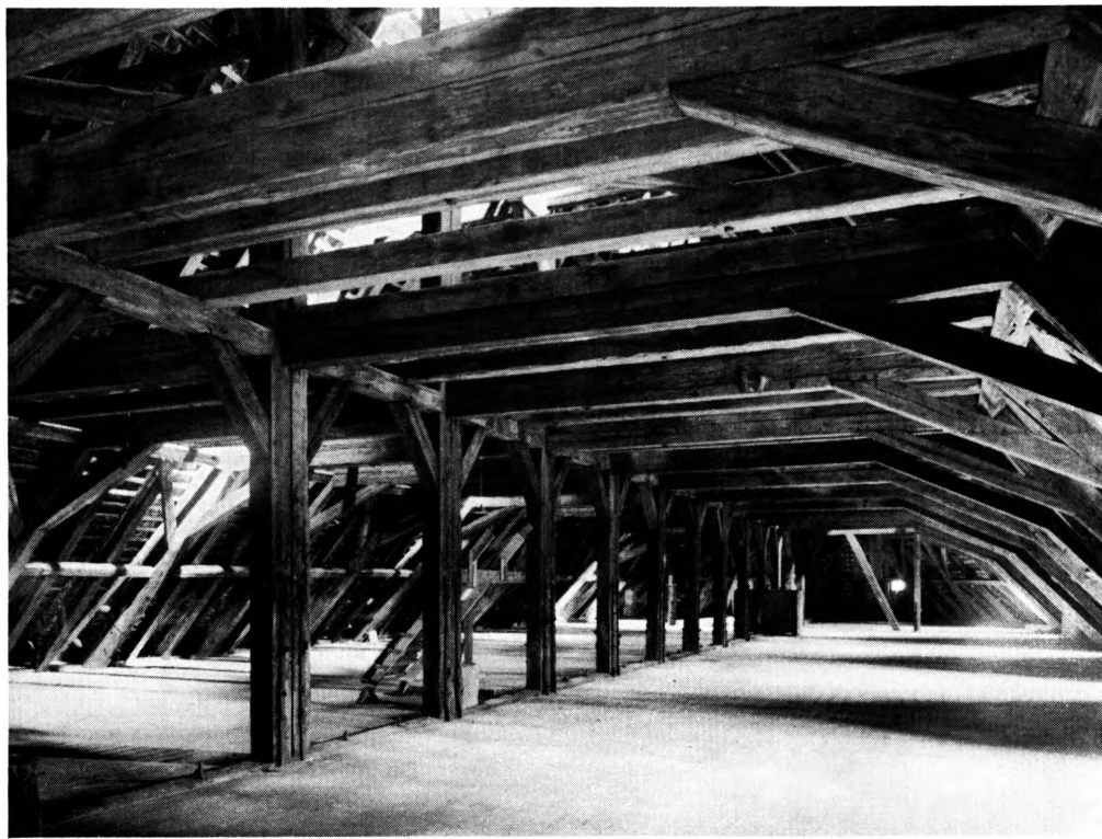
Fig. 22. Trinitatis kirke. Tagkonstruktionen, kaldet »Ringerloftet«.
