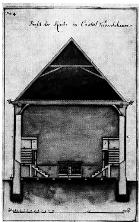
Fig. 7. Udkast til Kastelskirkens omdannelse 1696. Snit. Rigsarkivet.
