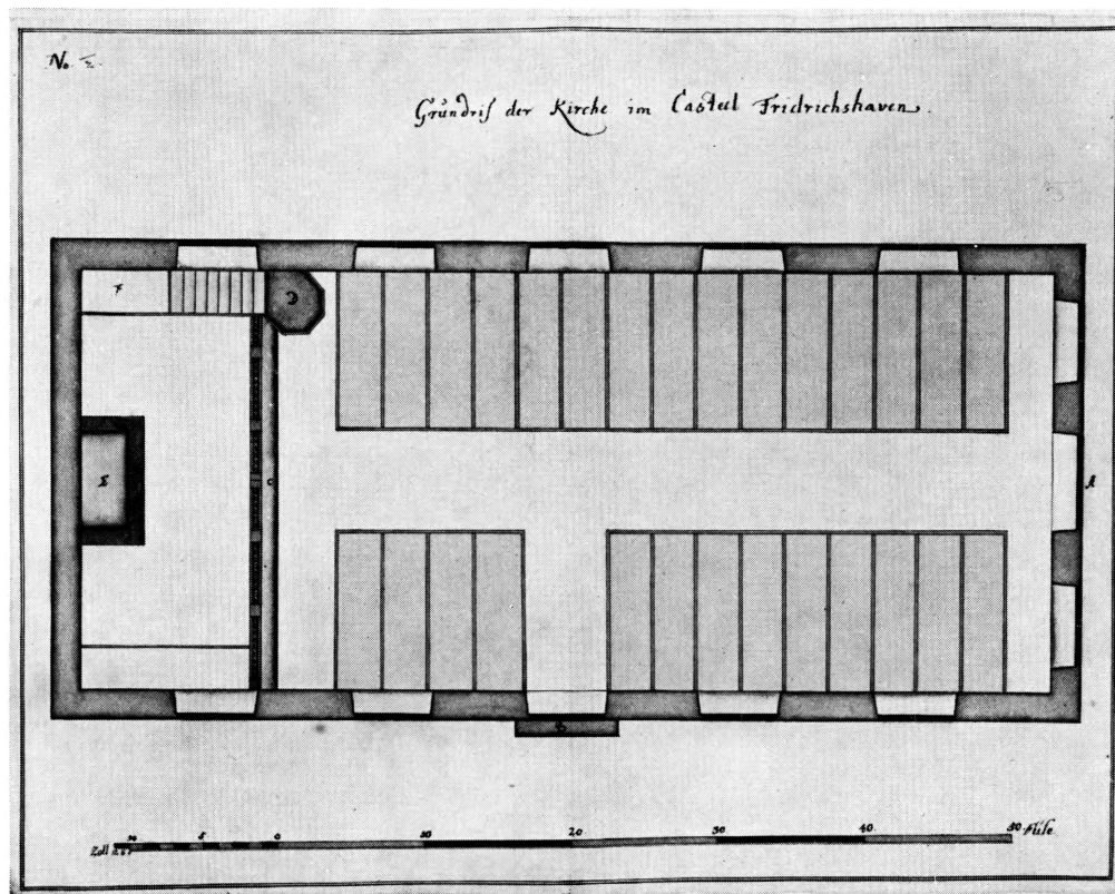
Fig. 5. Udkast til Kastelskirkens omdannelse 1696. Grundplan, vest opad. Rigsarkivet.
