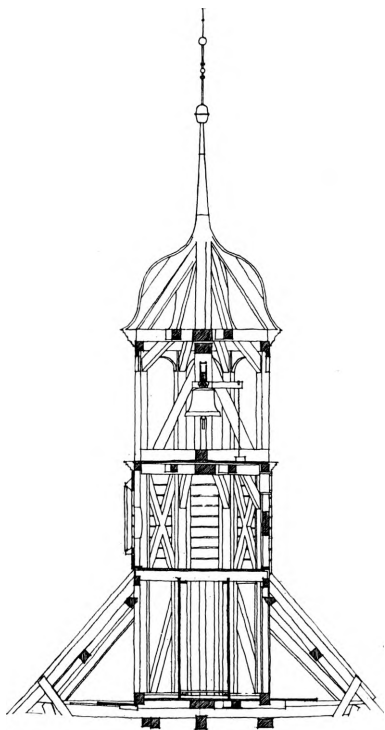
Fig. 24. Kastelskirken. Snit gennem tagrytteren.
