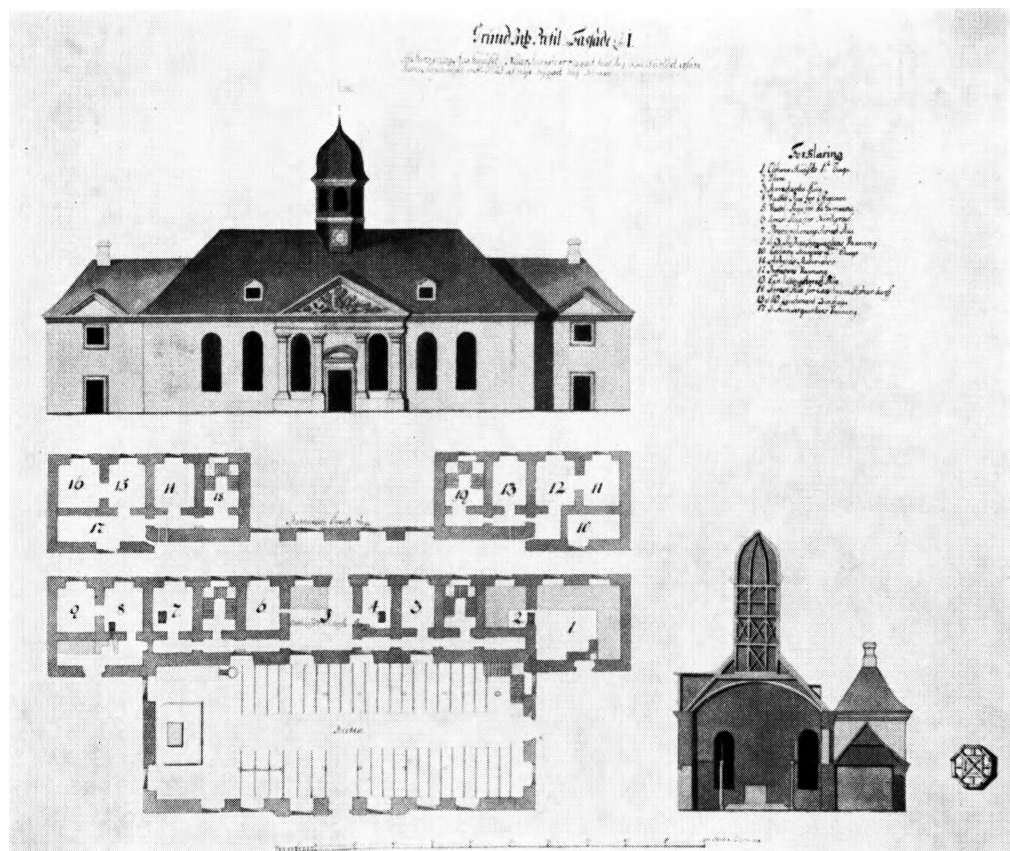
Fig. 9. Chr. Geddes opmåling af Kastelskirken 1754. Forsvarets Bygningstjeneste, historisk tegningsarkiv.
