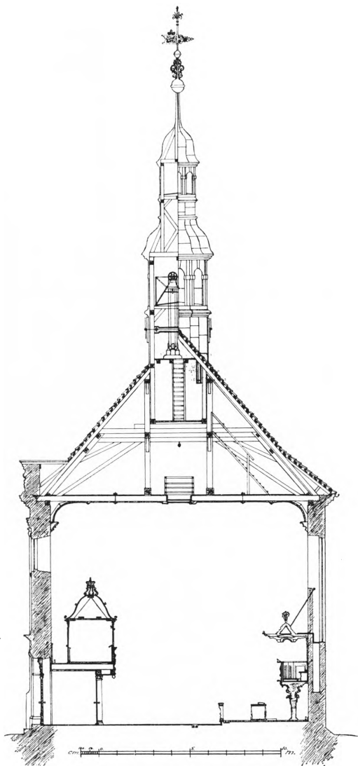
Fig. 13. Reformert kirke. Tværsnit opmålt o. 1920 af S. A. Junglov.
