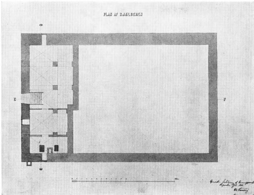
Fig. 11. Reformert kirkes krypt. Opmåling af Chr. Ramsing 1882 i kirkens sakristi.
