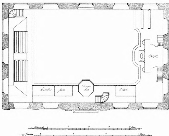
Fig. 7. Reformert kirke. Grundplan af pulpiturstokværk, målt 1914 af Alf. Jørgensen.
