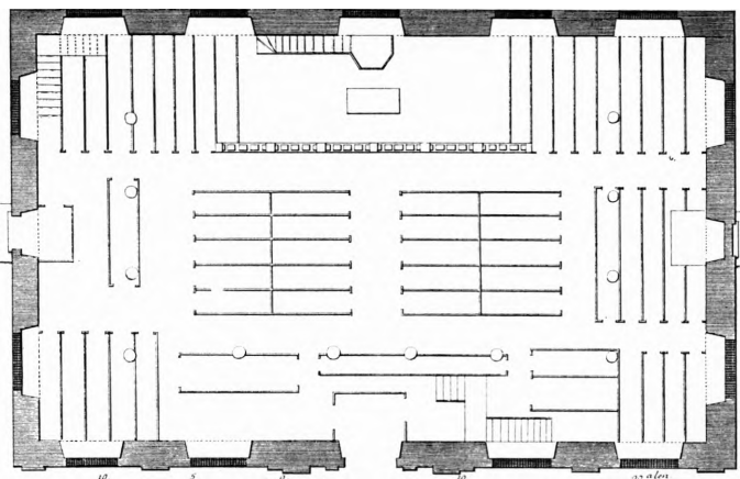
Fig. 35. Reformert kirke. Grundplan 1746 efter Danske Vitruvius.
