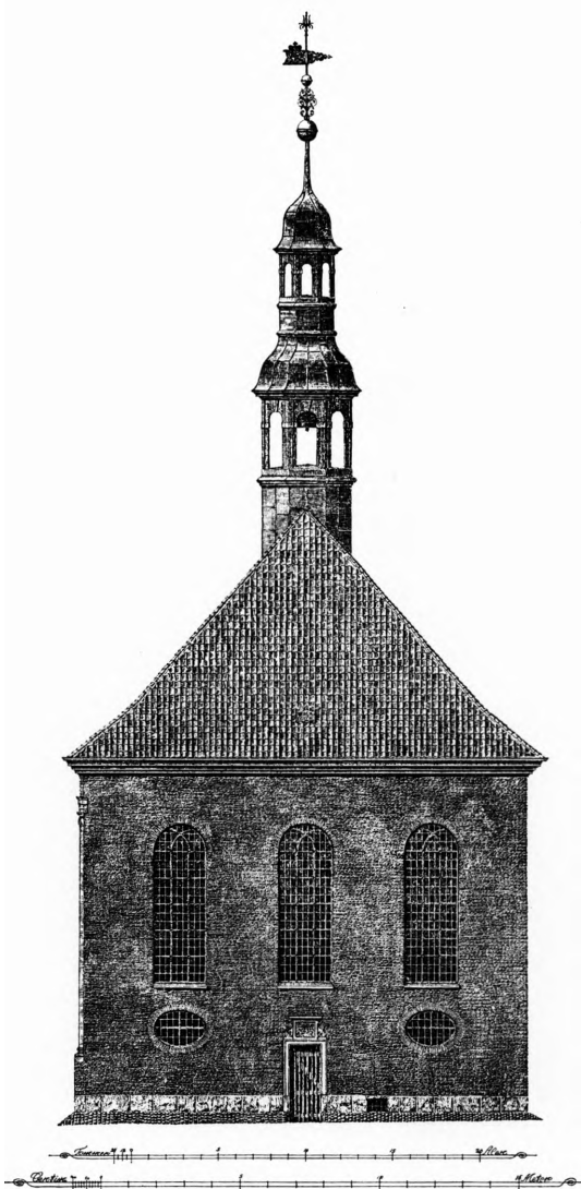
Fig. 9. Reformert kirke. Opstalt af gavl 1914, opmålt af Alf. Jørgensen.
