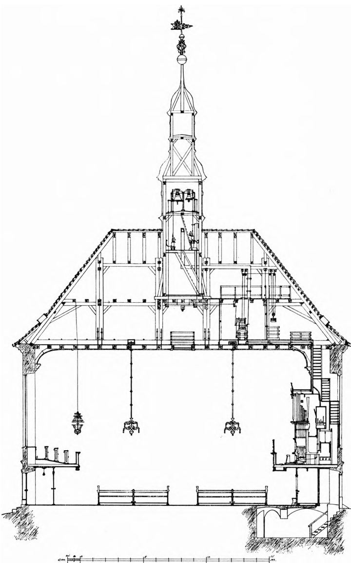
Fig. 12. Reformert kirke. Længdesnit opmålt o. 1920 af S. A. Jungløv.
