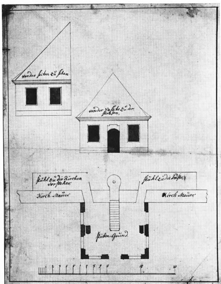
Fig. 38. Reformert kirke. Tegninger af et ikke udført sakristi o. 1770. (s. 64.) I det tyske arkiv.
