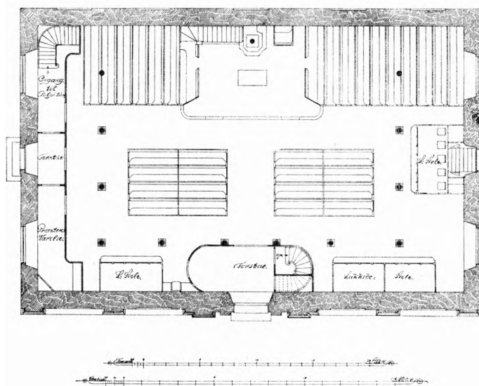
Fig. 6. Reformert kirke. Grundplan 1914, opmålt af Alf. Jørgensen.
