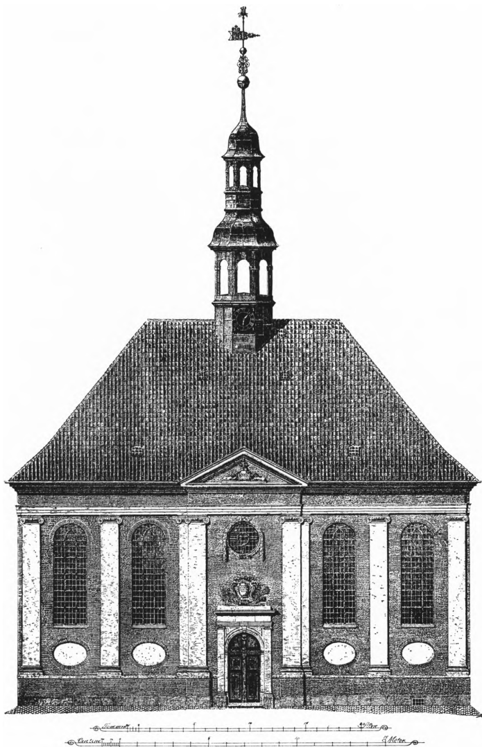
Fig. 8. Reformert kirke. Opstalt af façaden 1914, opmålt af Alf. Jorgensen.
