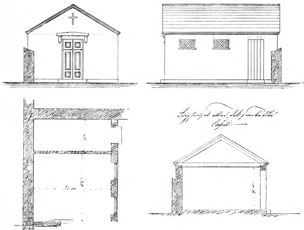
Fig. 65. Frederiksberg kirkegård. Lighus o. 1855. Usigneret tegning i LA (s. 482). Frederiksberg kirkeinspektionsarkiv.
