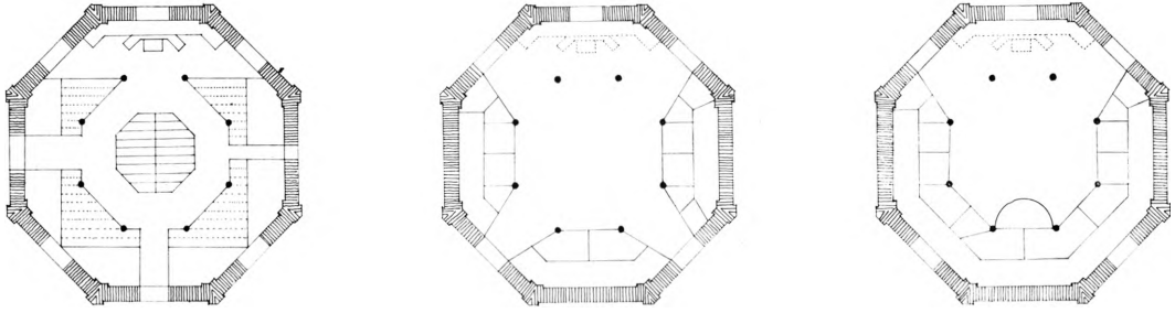
Fig. 23—25. Frederiksberg kirke. De forskellige stolestade- og pulpiturplaner, der er antydnet fig. 22, løst ud fra hinanden. Tilvenstre (fig. 23) gulvets plan, med tilføjelse af enkeltheder vedr. den rene ottekant, hentet fra ældre arkivalier (jfr. s. 454). — I midten (fig. 24) plan af det nederste pulpitur. — Til højre (fig. 25) plan af det midterste pulpitur. Planerne er udredet af Allan Tønnesen. Tegnet af Monica Thon efter forfatterens direktiver.
