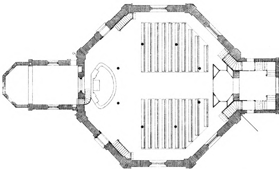
Fig. 9—10. Frederiksberg kirke, opmålt 1912 af A. Glahn. 1: 300. Foroven (fig. 9) opstalt af nordsiden. Forneden (fig. 10) plan af gulvet; syd opad.
