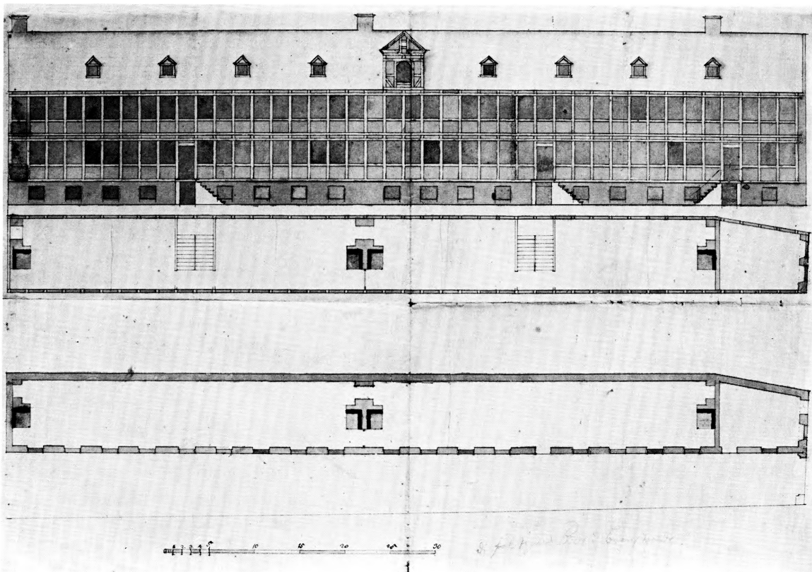
Fig. 135. Facade og planer til sidehuset 1731 (?). 1:400 (s. 155). RA. – Facade and plans for the side-house 1731(?)
