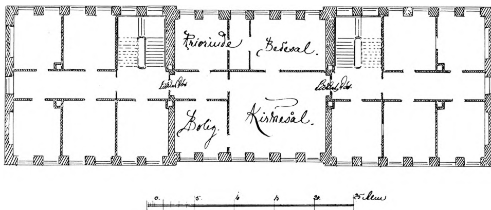
Fig. 169. Etageplan af første sal ved A. Møller 1874 (s. 188). 1:300. Københavns bolig- og byggedirektorat. – Floor plan of the first floor by
