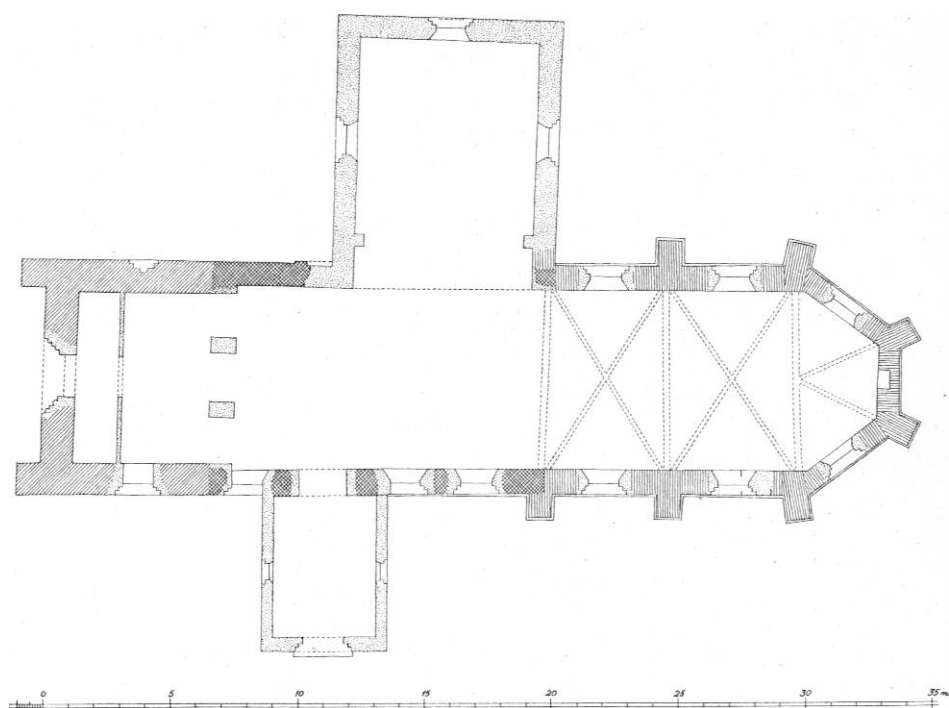
Fig. 3. Rødby. Plan. 1:300. Målt af Kunstakademiets bygningsskole 1944.
