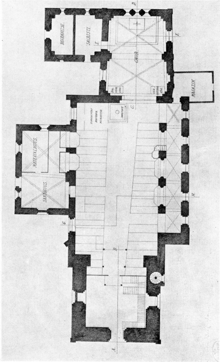
Fig. 10. Stubbekøbing. Plan for restaureringen. 1:300, Målt af V. Tvede 1861.
