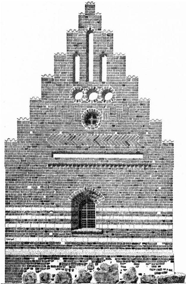
Fig. 11. Stubbekøbing. Østgavl af S. Annas kapel. 1:100. Målt af Vagn Thorborg 1943 (s. 263).
