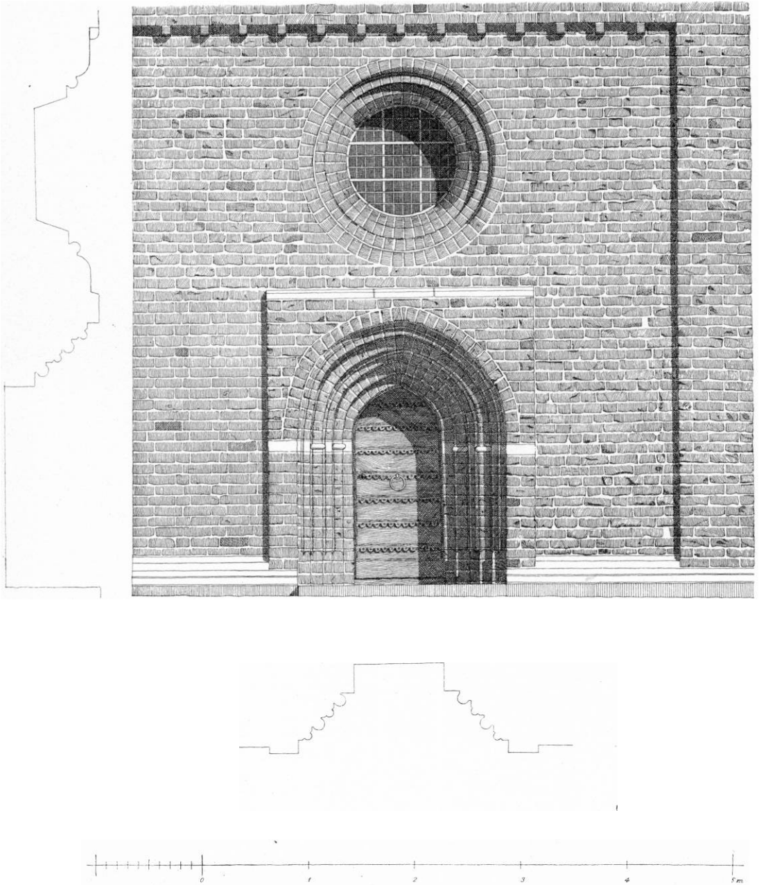
Fig. 8. Stubbekøbing. Dør på korets sydside. 1:50. Det runde vindue er moderne. Målt af Erik Glud 1943 (s. 261).
