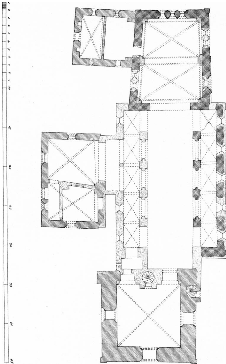
Fig. 3. Stubbekøbing. Plan. 1:300. Øst opad. Målt af J. Thomsen 1943.
