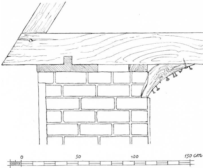
Fig. 4. Gloslunde. Tagfoden over skibet med murlægte og konsol for skibets hulkehl under loftet. 1:20. Målt af M. Clemmensen 1914.
