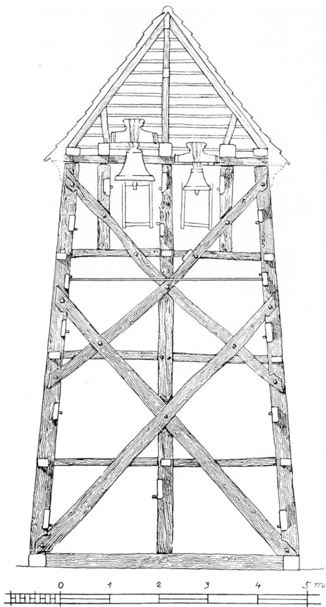
Fig. 6. Gloslunde. Klokkestabel. Snit. 1:75. Målt af M. Clemmensen 1914.
