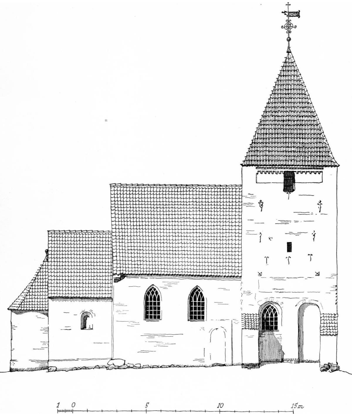
Fig. 3. Ryde. Kirkens nordside. 1:150. Målt af Mogens Clemmensen o.1915.
