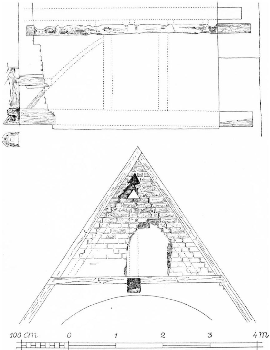
Fig. 5. Ryde. Korets tagkonstruktion. 1:50. Øverst set fra nord, nederst set mod vest. Målt af M. Clemmensen 1919.
