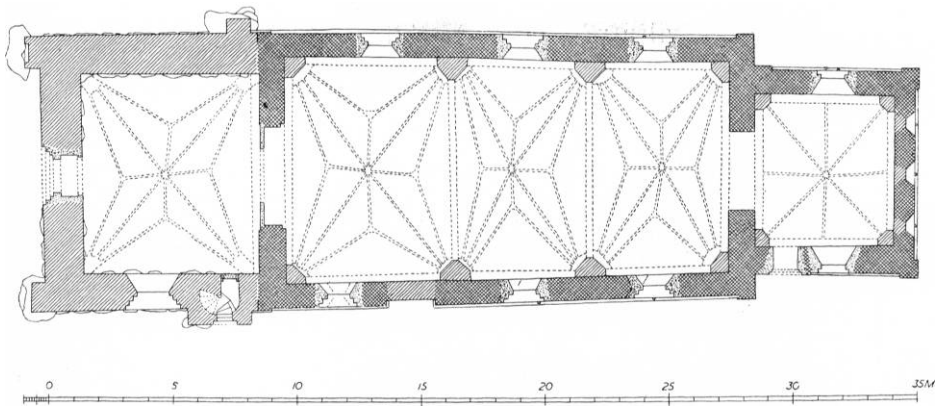
Fig. 2. Købelev. Plan. 1:300. Målt af Volmer Hoffmeyer 1941.
