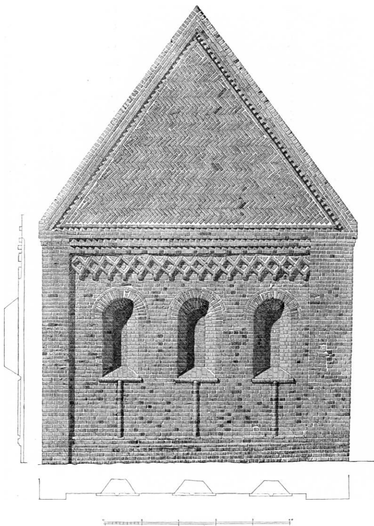
Fig. 3. Købelev. Korets ostgavl. 1:100. Målt af Charles Christensen 1950 (s. 499).
