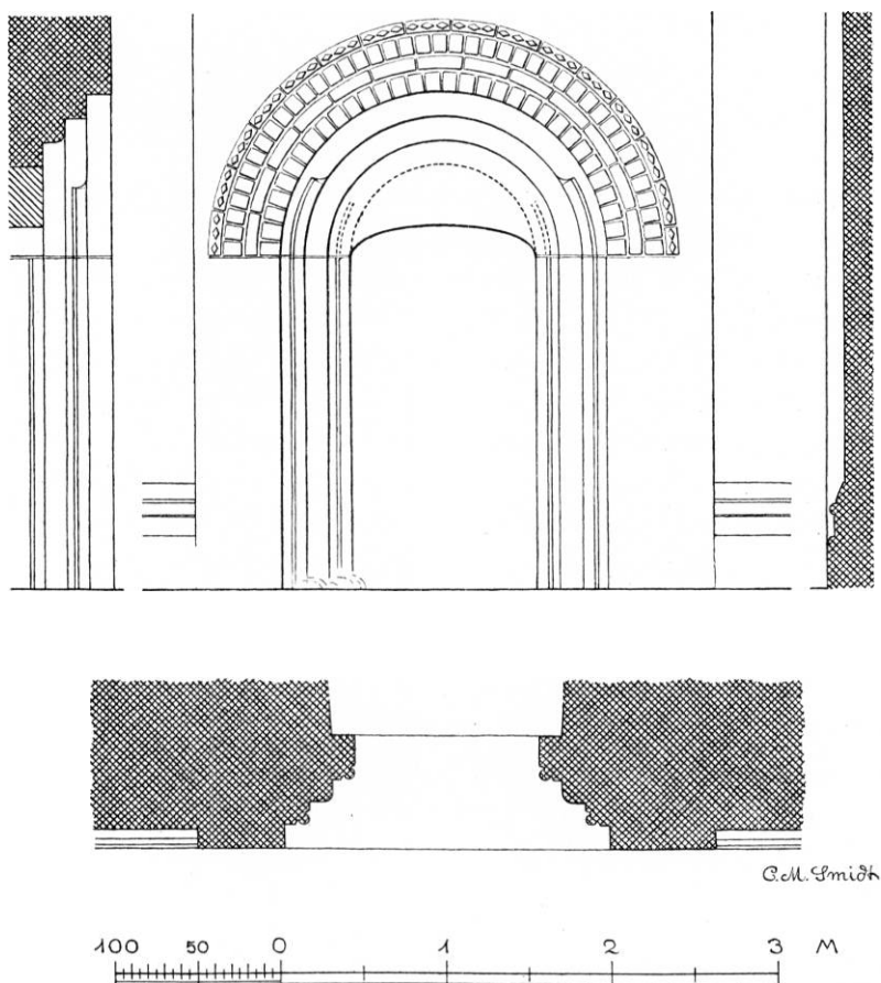
Fig. 4. Vindeby. Skibets sydportal. 1:50. Målt af C. M. Smidt 1934 (s. 517).
