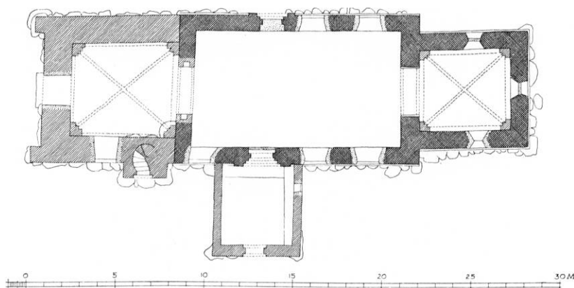
Fig. 2. Vindeby. Plan. 1:300. Målt af Charles Christensen 1950.
