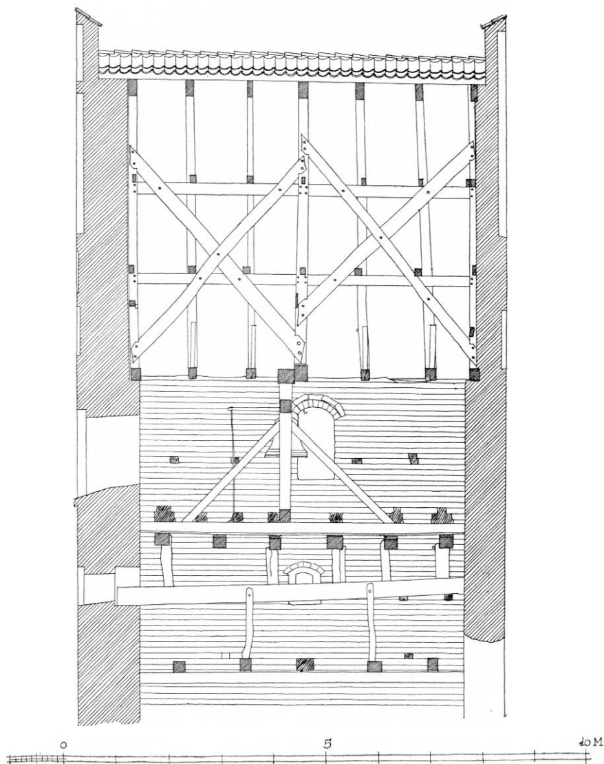
Fig. 6—7. Vindeby. Snit vest-øst af tårnets øvre stokværk og nord-syd af hele tårnet. 1:100. Målt af Edvard Vollquarts 1942.
