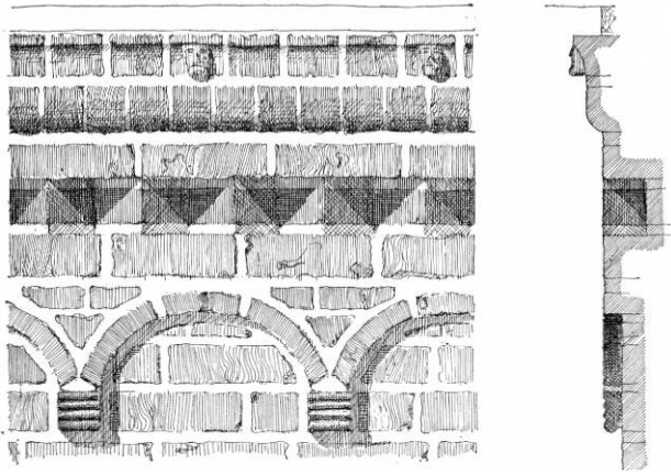
Fig. 4. Utterslev. Gesims på korets sydside. 1:5. Målt af Jens Sidenius 1942 (s. 533).
