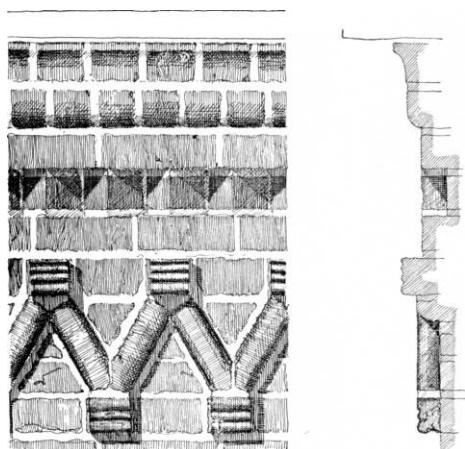
Fig. 5. Utterslev. Gesims på korets nordside. 1:5. Målt af Jens Sidenius 1942 (s. 533).
