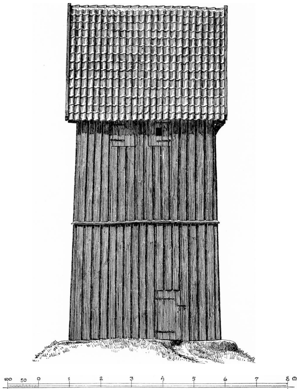
Fig. 5. Birket. Klokkestabelens sydside. 1:75. Målt af Mogens Clemmensen 1909 (s. 640).
