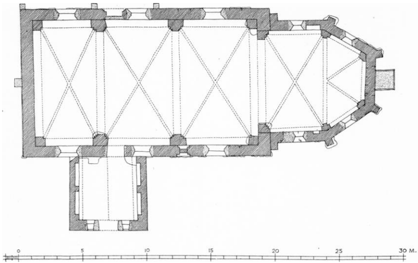
Fig. 2. Birket. Plan. 1:300. Målt af El. M. 1948.
