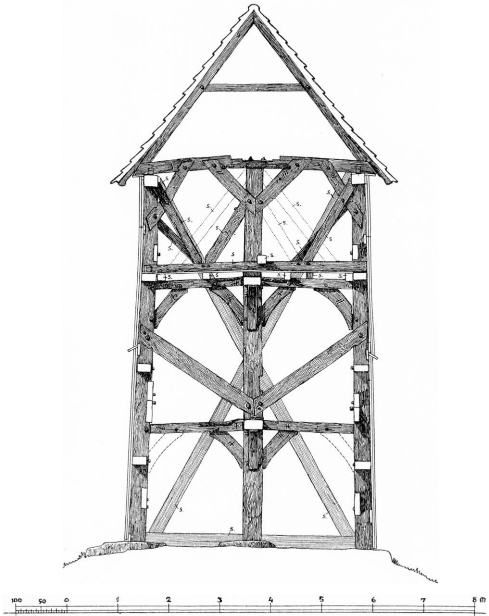
Fig. 6. Birket. Snit af klokkestabelen, set mod vest. 1:75. Målt af Mogens Clemmensen 1909. S = senere indsatte afstivninger (s. 640).
