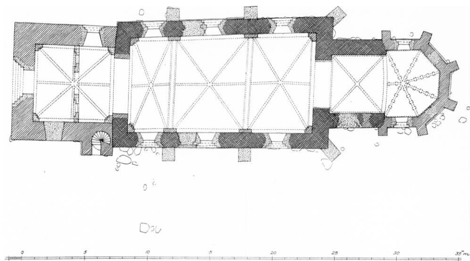
Fig. 2. Erindlev. Plan. 1:300. Målt af Grethe Kølle 1948.
