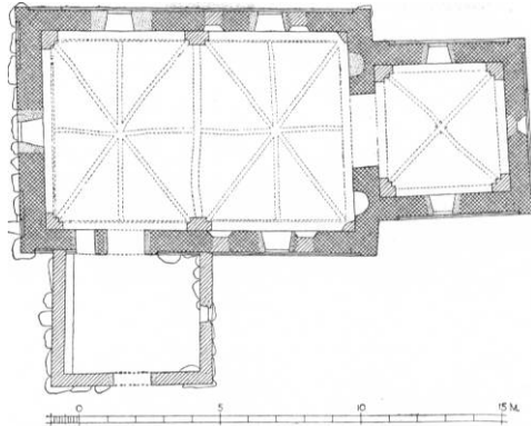
Fig. 2. Nebbelunde. Plan. 1:300. Målt af Jarl Ove Skipper 1944.
