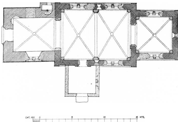
Fig. 2. Taars. Plan. 1:300. Målt af H. Schibbye 1942.
