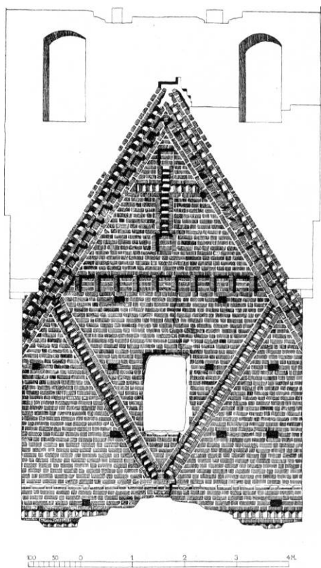
Fig. 6. Taars. Skibets vestgavl. 1:100. Målt af Jørgen Buchardt-Larsen 1942.
