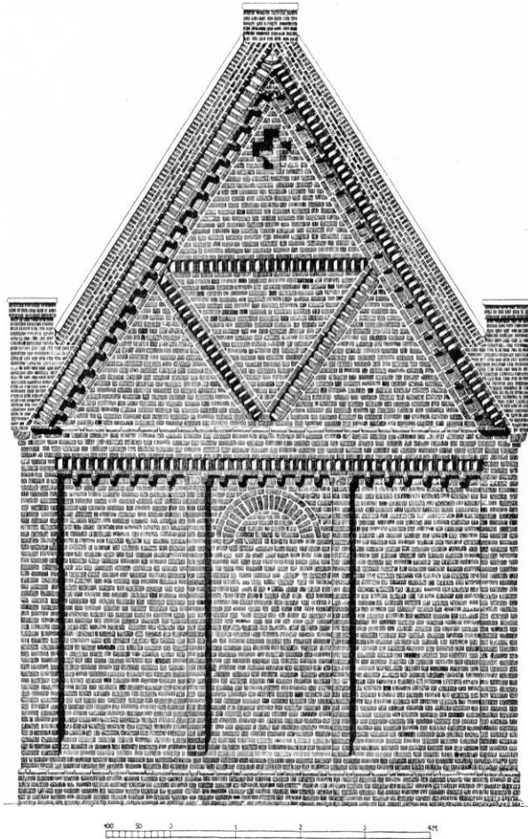
Fig. 3. Taars. Korets østgavl. 1:100. Målt af Jørgen Buchardt-Larsen 1942.
