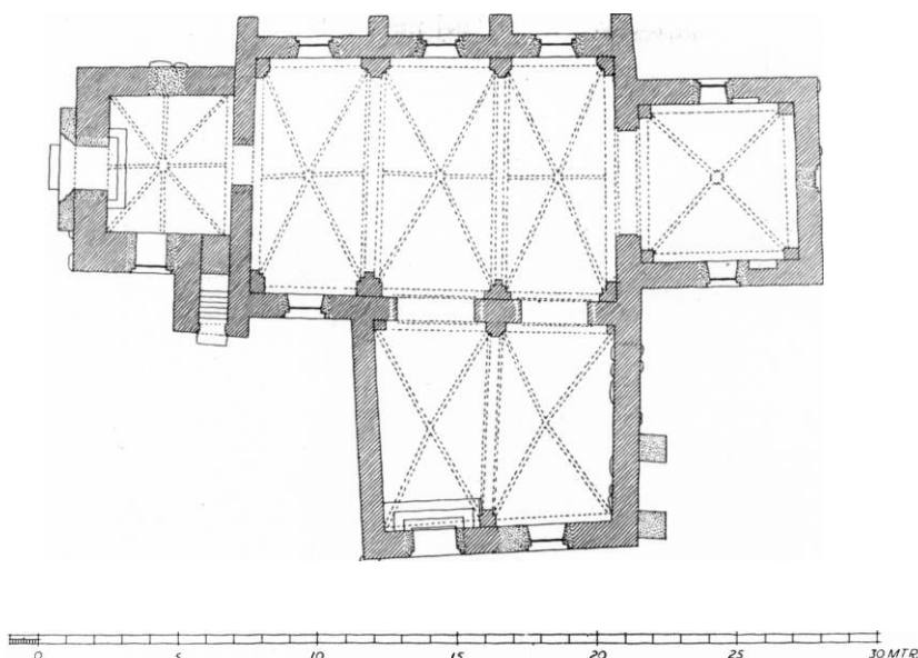
Fig. 2. Majbølle. Plan. 1:300. Målt af A. W. Fyhn 1951.
