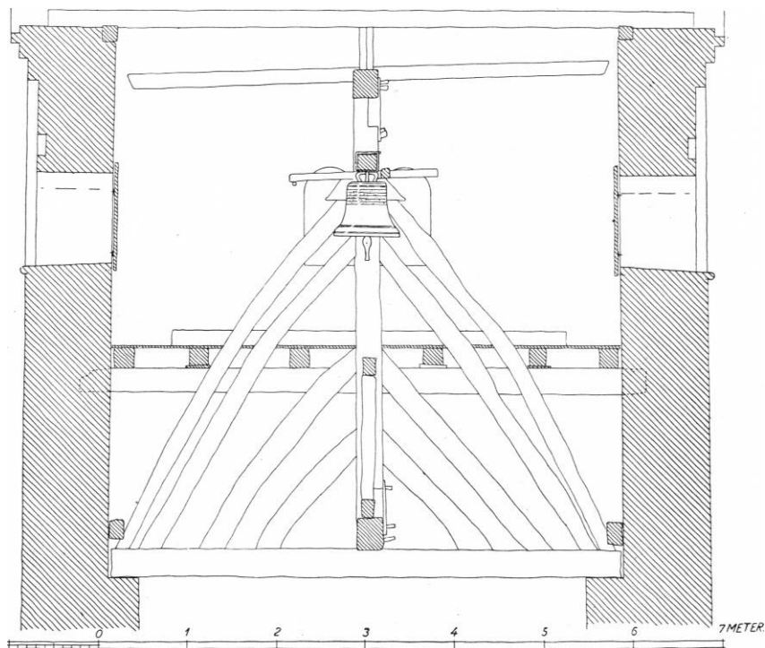
Fig. 6. Majbølle. Klokkestol. Snit nord—syd. Målt af A. W. Fyhn 1951 (s. 970).
