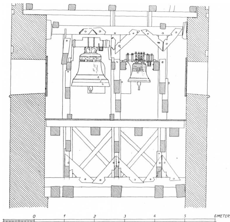
Fig. 5. Majbolle. Klokkestol. Snit vest—øst. Målt af A. W. Fyhn 1951 (s. 970).
