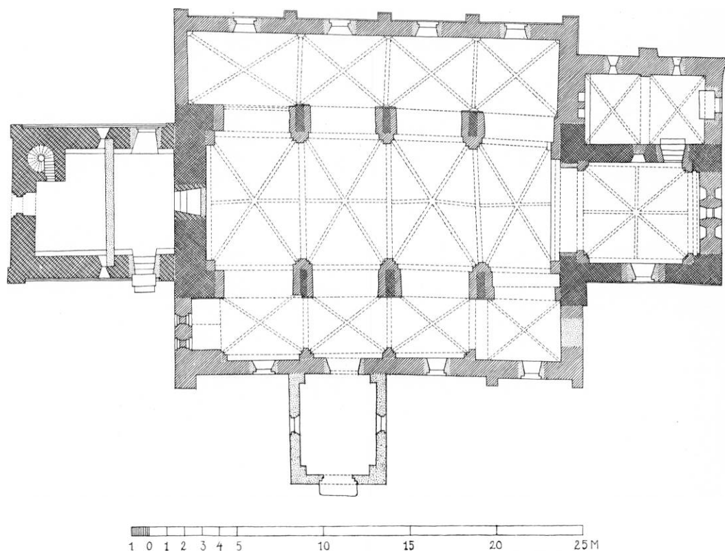
Fig. 2. Toreby. Plan. 1:300. Målt af Kunstakademiets arkitekturskole 1938.
