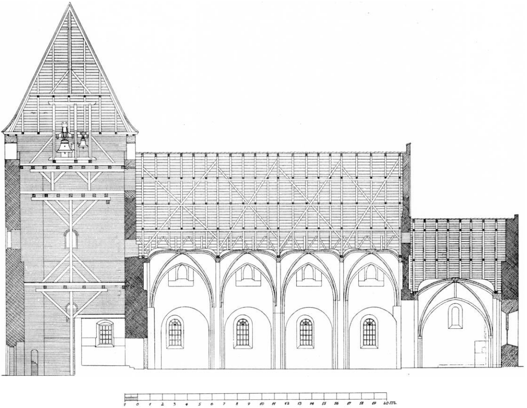
Fig. 5. Toreby. Langsnit. 1:300. Målt af Edvin Ravn 1938.
