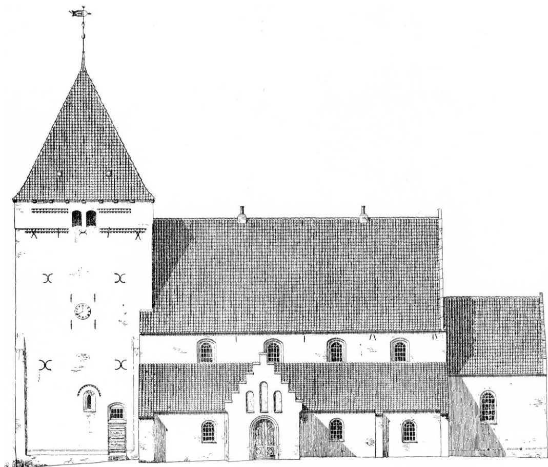
Fig. 3. Toreby. Sydfaçade. 1:300. Målt af Ørnsholt og Køhler 1910.
