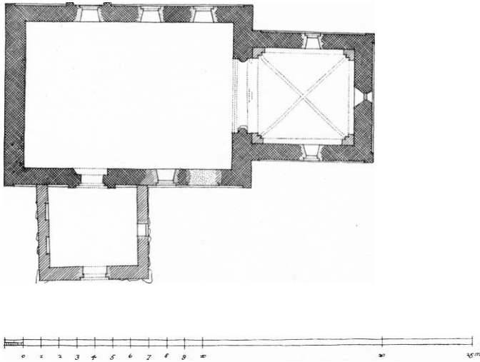
Fig. 2. Maglebrænde. Plan. 1:300. Målt af Erik Eriksen 1943.
