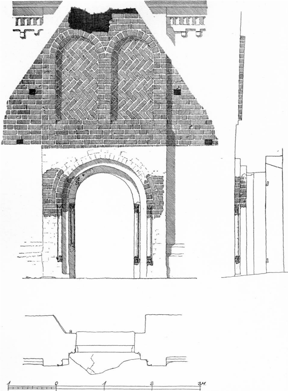
Fig. 4. Maglebrænde. Sydportal. 1:50. Målt af Ejler Rasmussen 1942 (s. 1119).
