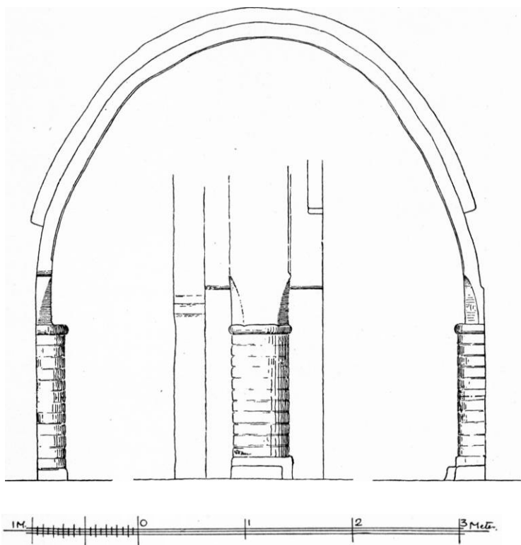
Fig. 5. Maglebrænde. Korbuen, set fra vest, med søndre vange, set fra nord, indsat. 1:50. Målt af C. Barfod 1911 (s. 1122).
