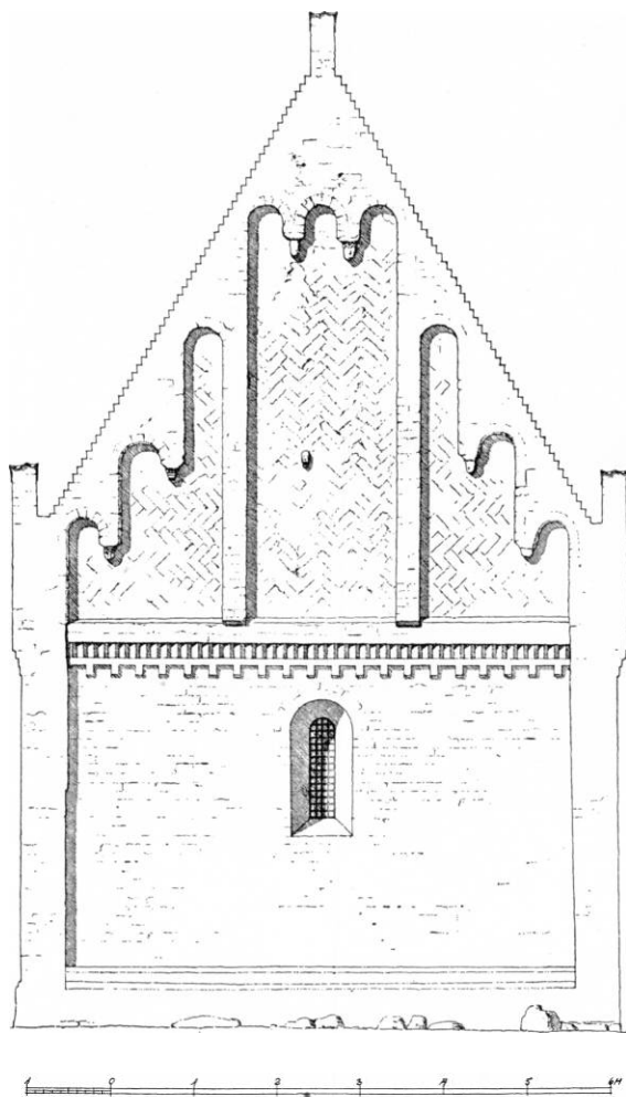
Fig. 3. Maglebrænde. Korets østgavl. 1:100. Målt af Ejler Rasmussen 1943 (s. 1118).
