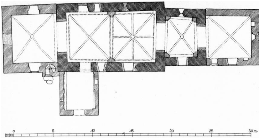
Fig. 2. Torkilstrup. Plan. 1:300. Målt af Aa. Rl. 1940.
