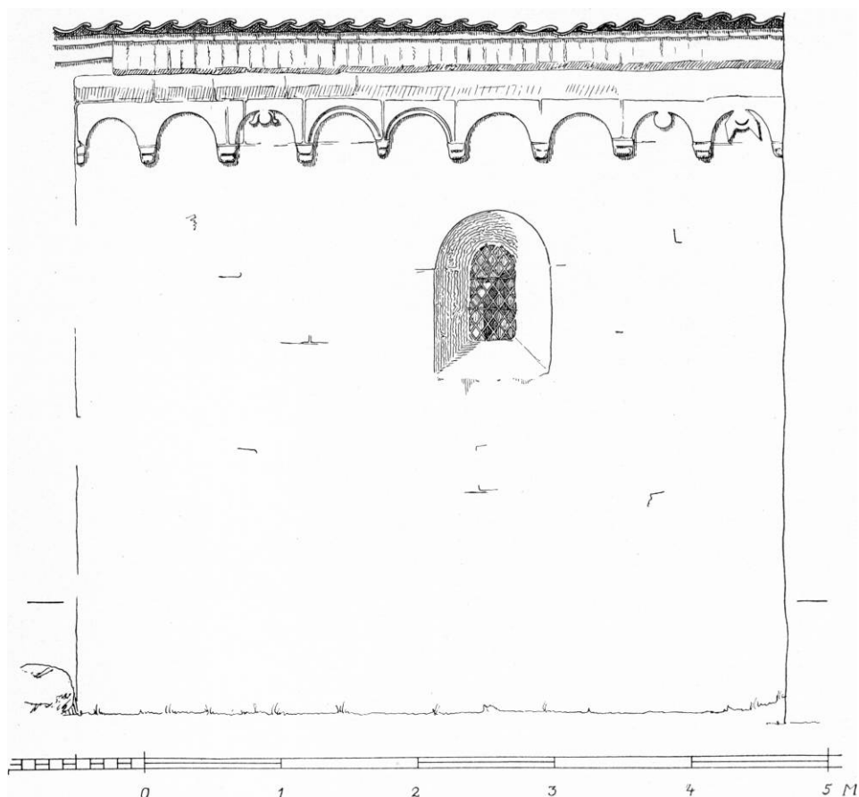
Fig. 4. Torkilstrup. Korets nordside. 1:50. Målt af Aa. RI. 1940 (s. 1131).
