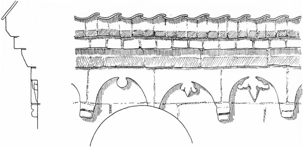
Fig. 3. Torkilstrup. Gesims på korets sydside. 1:20. Målt af Aa. Rl. 1940 (s. 1131).
