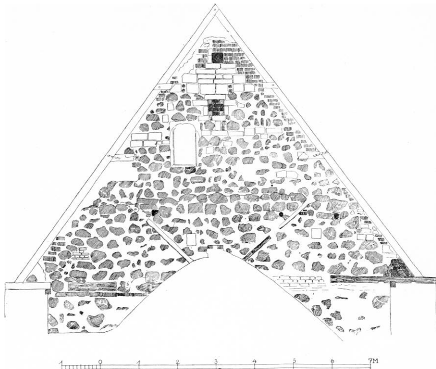
Fig. 4. Tingsted. Skibets vestgavl. 1:100. Målt af Helge Foss 1942 (s. 1311).
