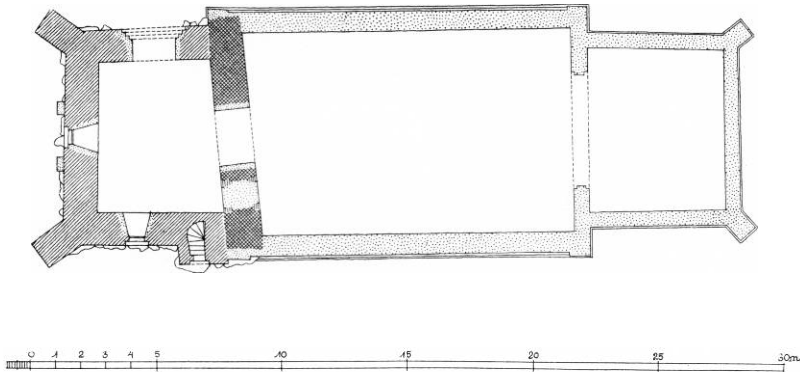
Fig. 2. Skelby. Plan. 1:300. Målt af Tove Bojesen 1953.
