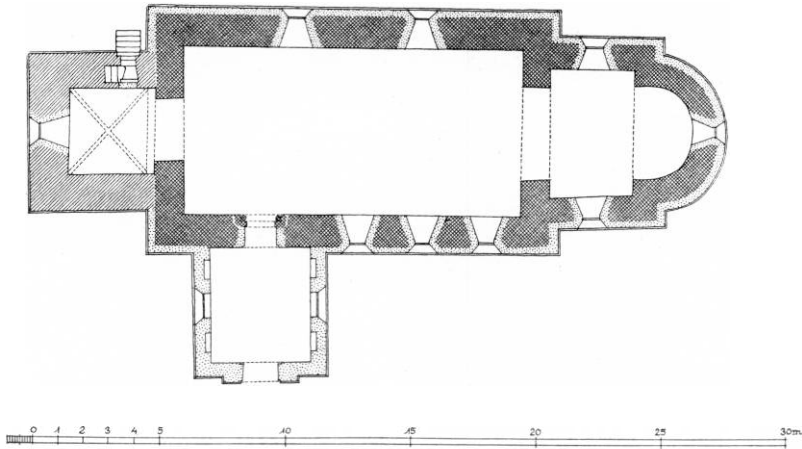
Fig. 2. Sdr. Kirkeby. Plan. 1:300. Målt af Tove Bojesen 1953.
