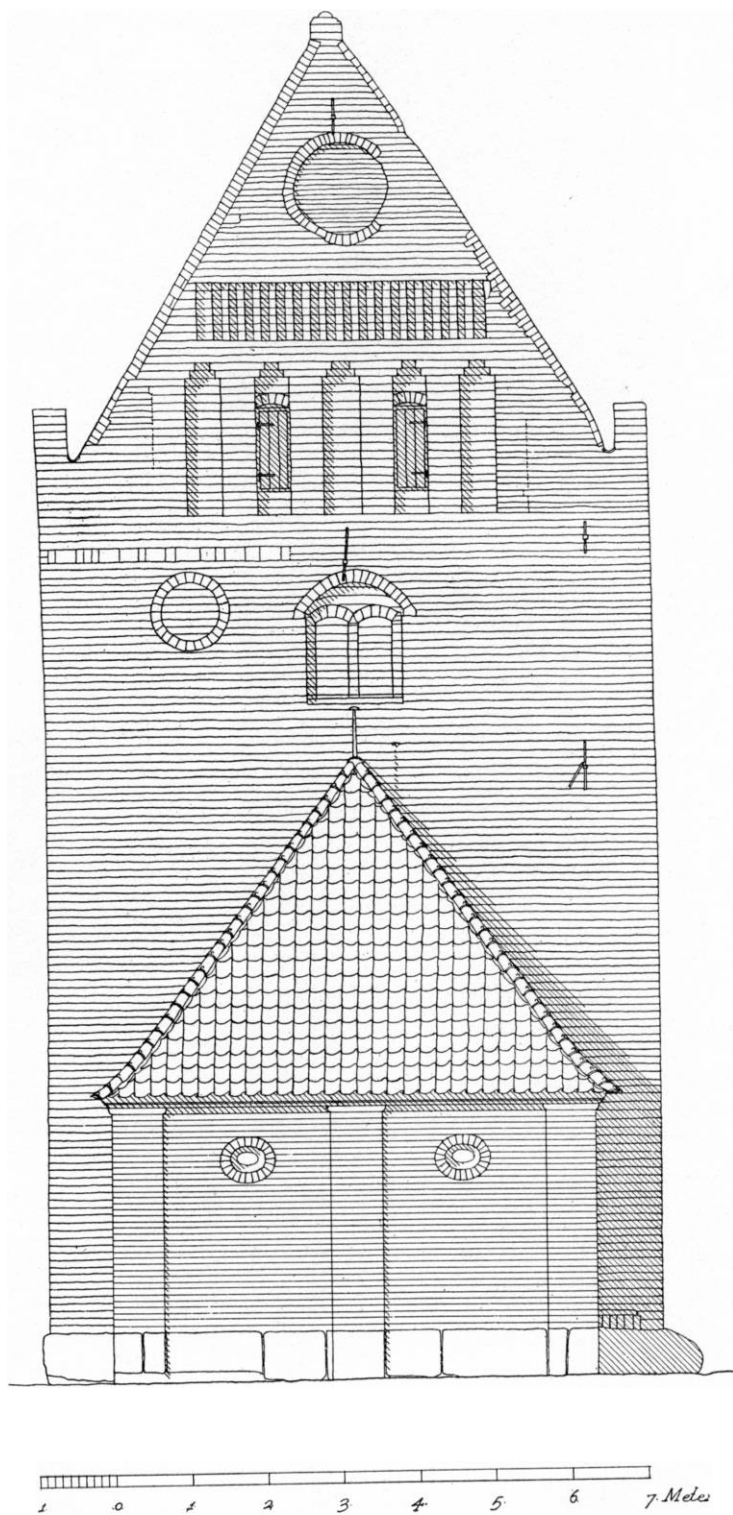
Fig. 4. Sdr. Alslev. Vestfaçade. 1:100. Målt af H. Gyrsting Hansen 1942.
