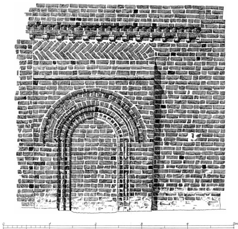
Fig. 3. Sdr. Alslev. Nordportal. 1:50. Målt af Ib Husted Jørgensen 1942.
